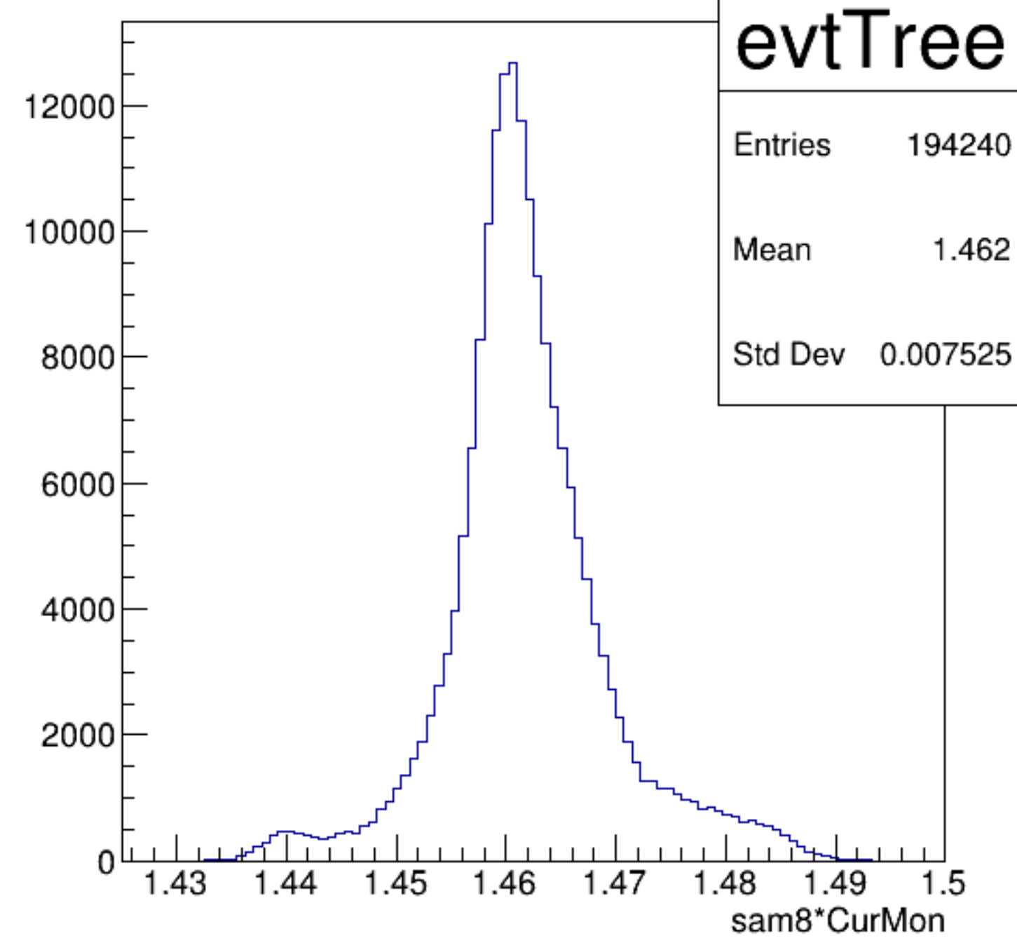
sam8*CurMon {ErrorFlag==0}
