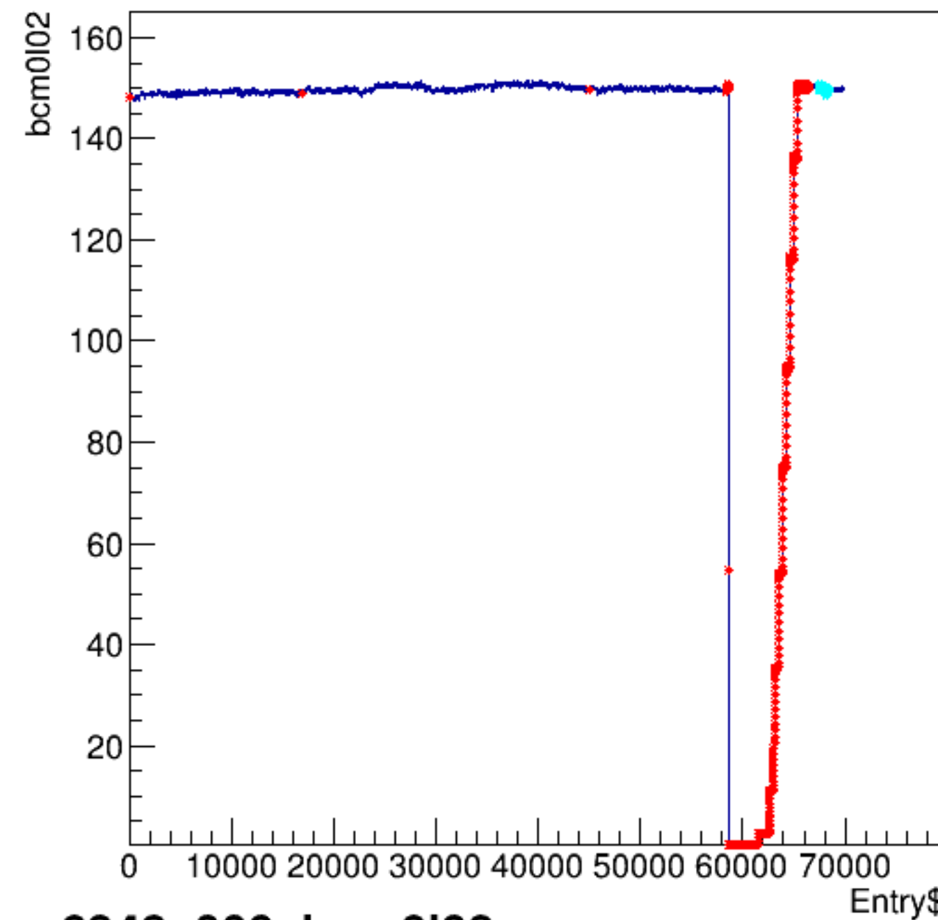
bcm0l02:Entry$
