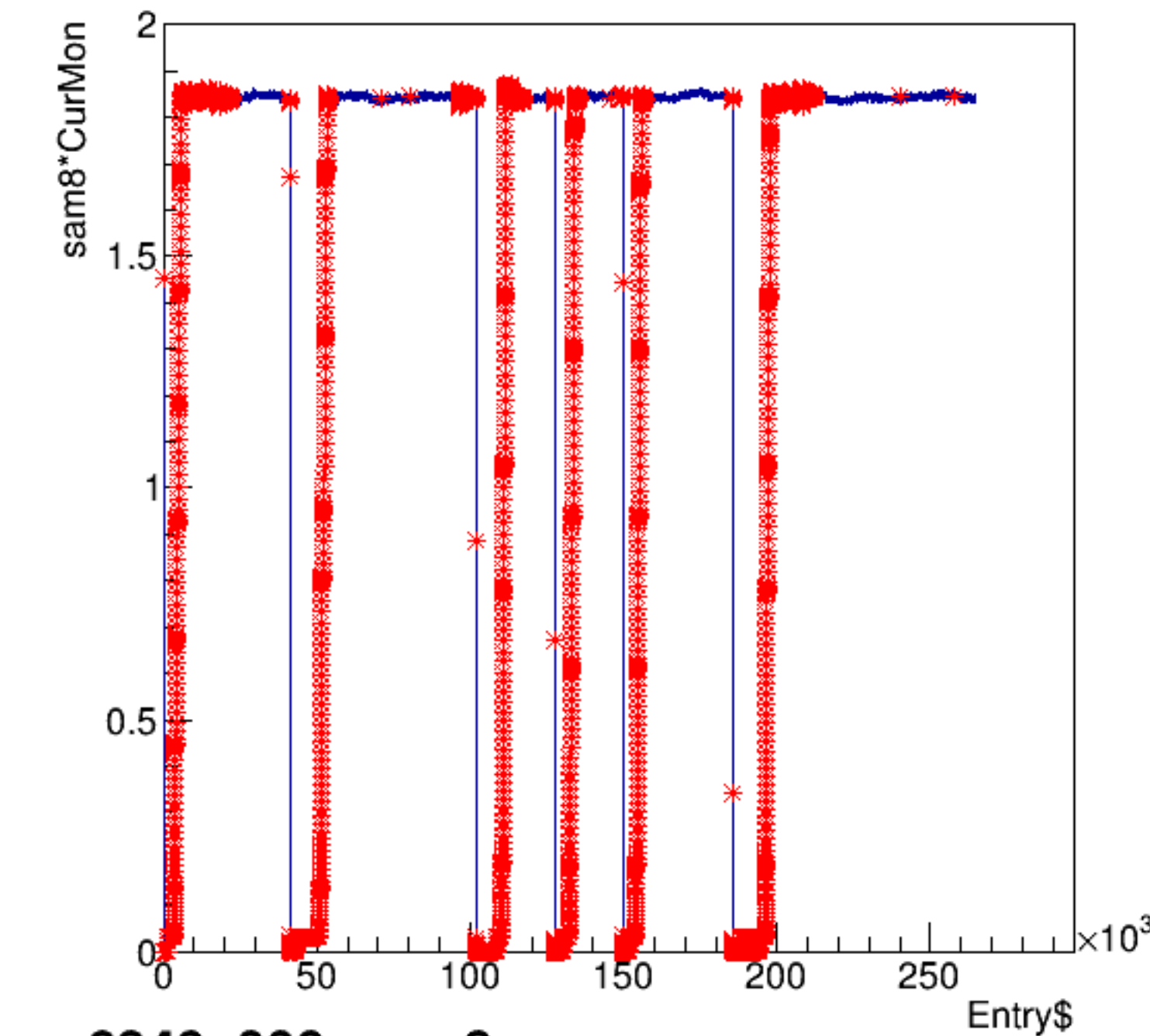
sam8*CurMon:Entry$
