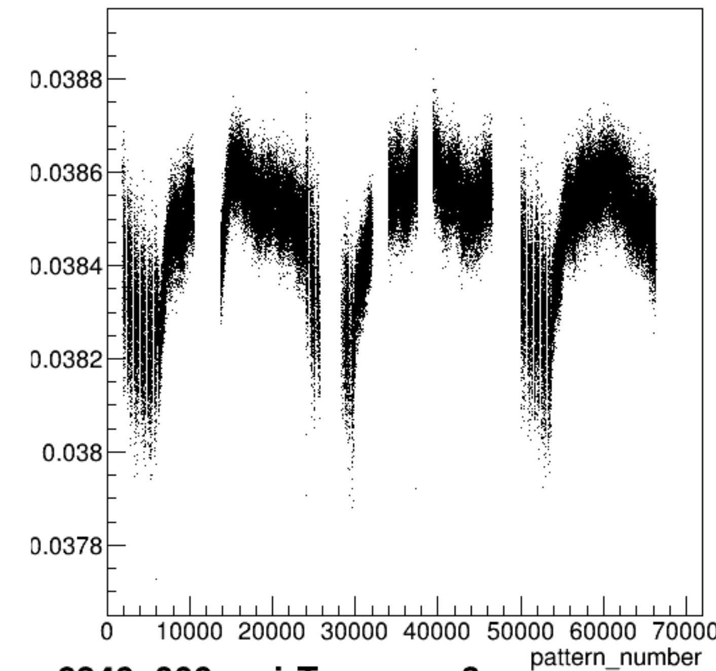
yield_sam3:pattern_number {ErrorFlag==0}
