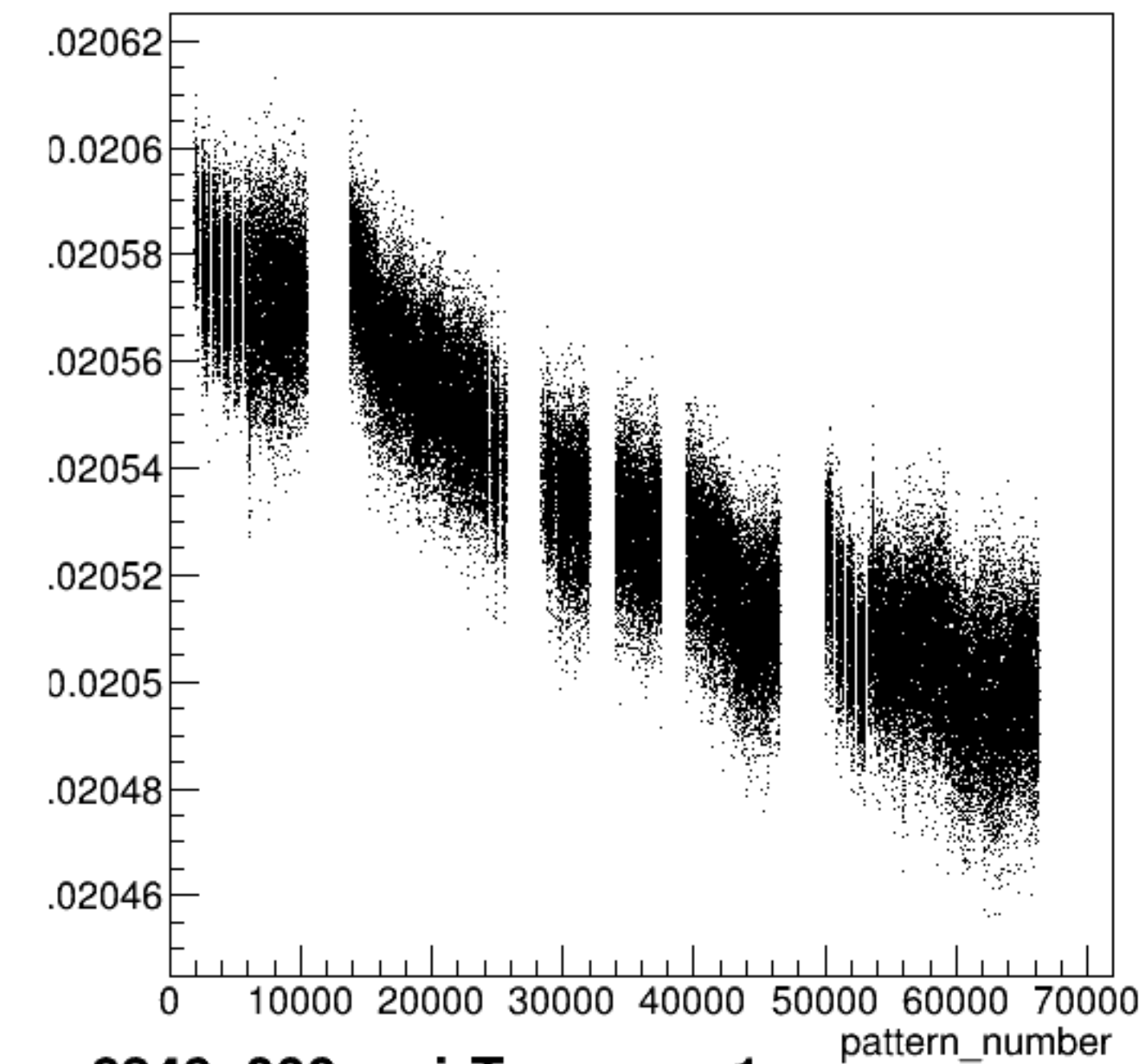
yield_sam1:pattern_number {ErrorFlag==0}
