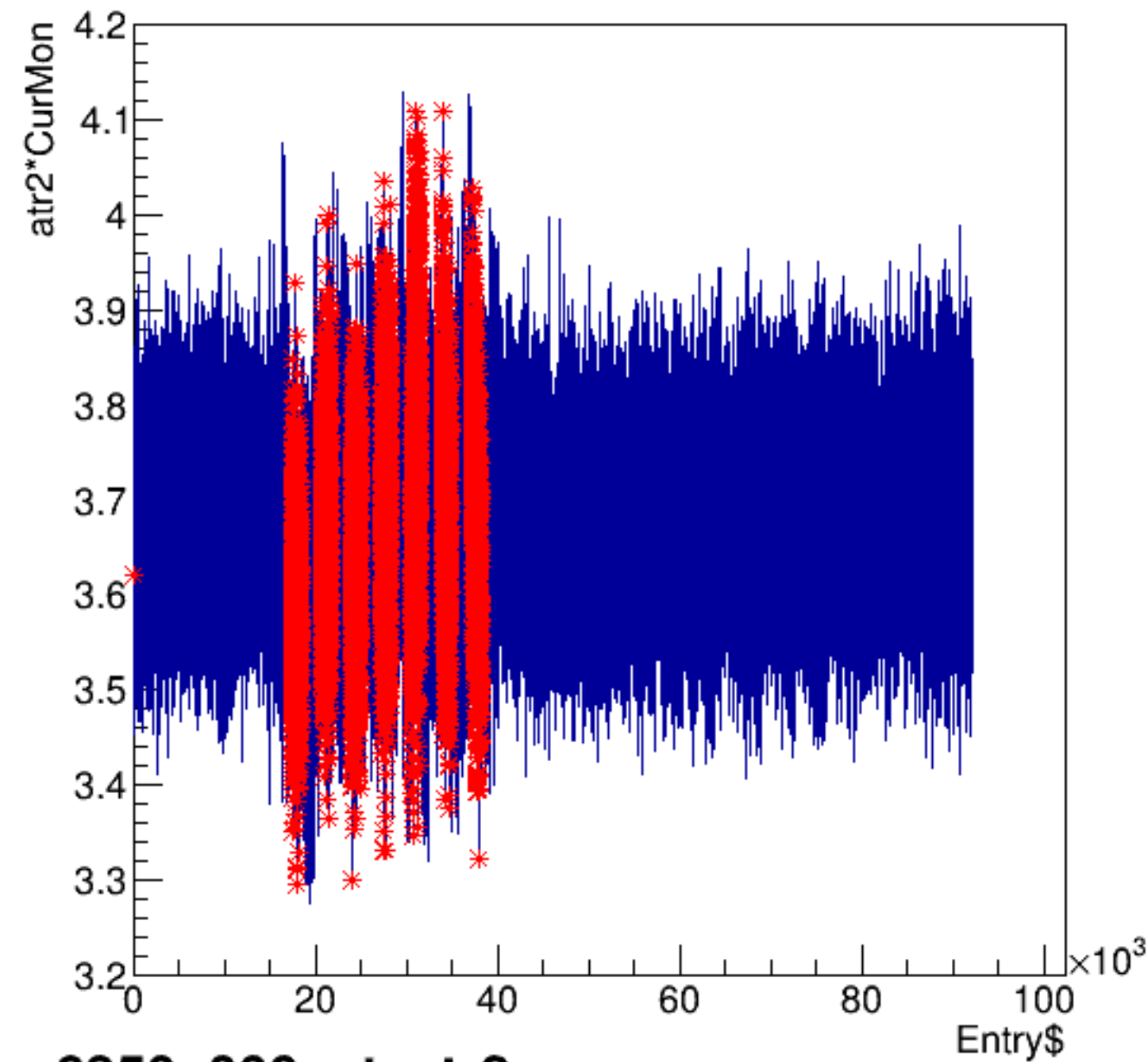
atr2*CurMon:Entry$
