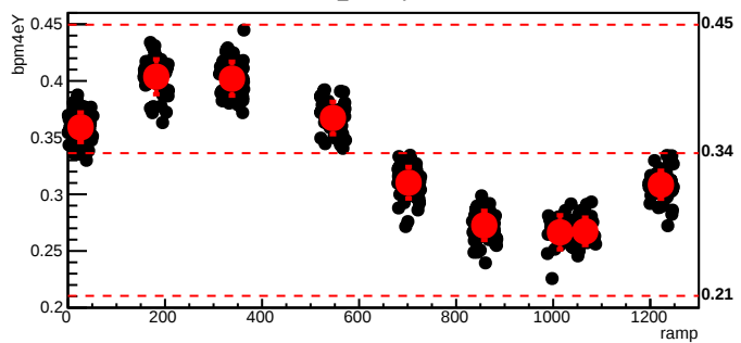
bmod_trim2,cyc=6030
