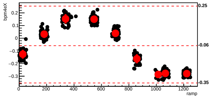
bmod_trim5,cyc=6030
