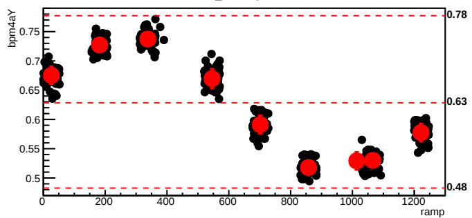
bmod_trim4,cyc=6030
