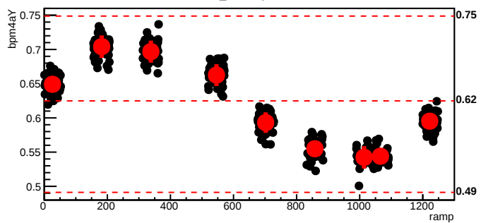
bmod_trim2,cyc=6030
