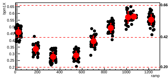
bmod_trim3,cyc=6033
