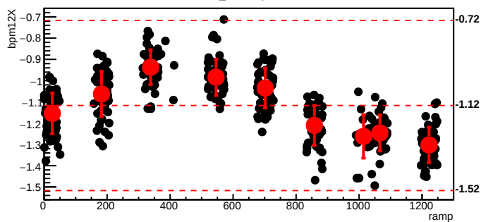
bmod_trim5,cyc=6033
