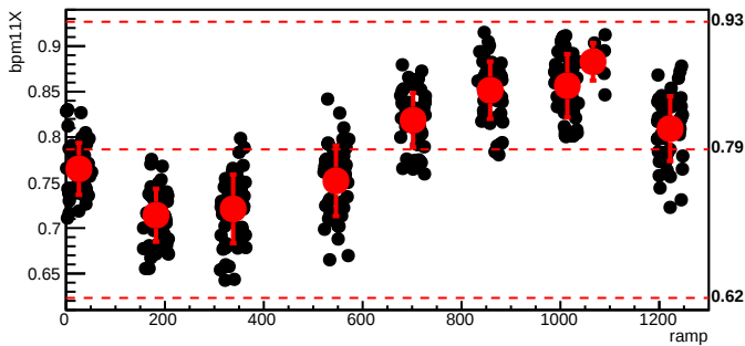
bmod_trim7,cyc=6033
