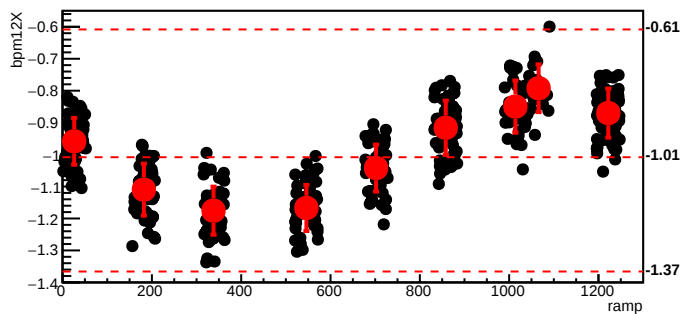
bmod_trim3,cyc=6033
