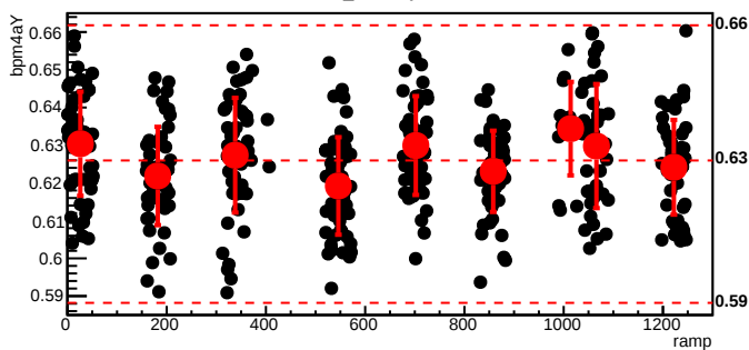
bmod_trim5,cyc=6033
