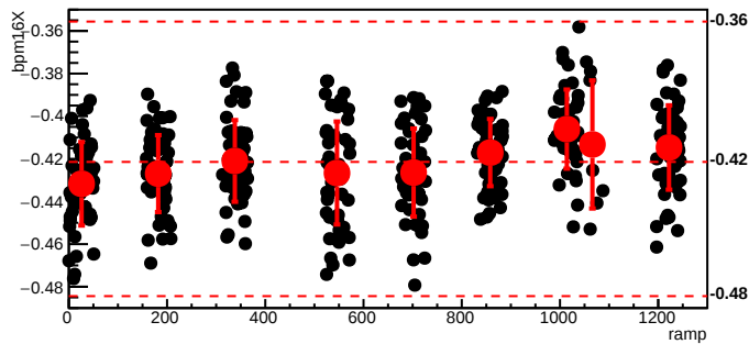
bmod_trim7,cyc=6033
