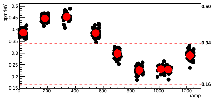
bmod_trim4,cyc=6033
