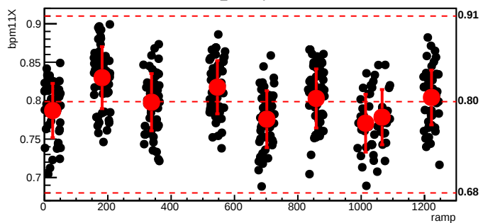
bmod_trim6,cyc=6033
