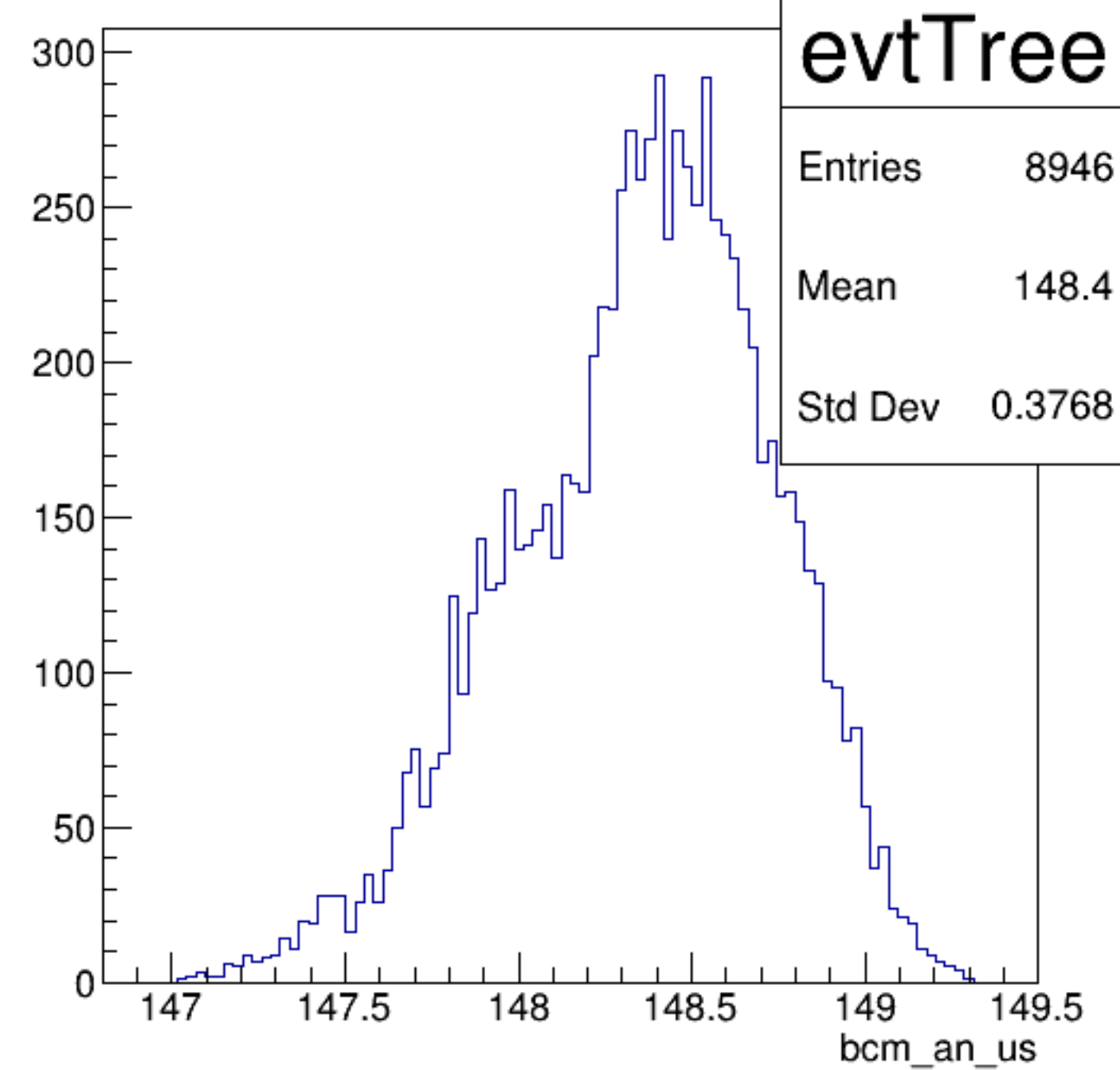
bcm_an_us {ErrorFlag==0}
