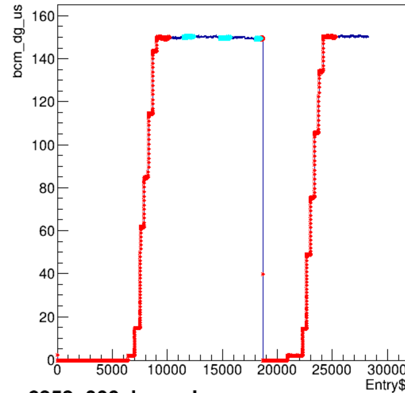
bcm_dg_us:Entry$
