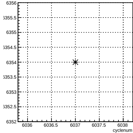
run:cyclenum {run == 6354}
