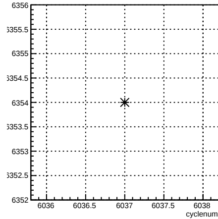
run:cyclenum {run == 6354}
