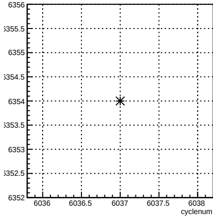
run:cyclenum {run == 6354}
