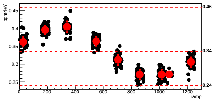
bmod_trim2,cyc=6041
