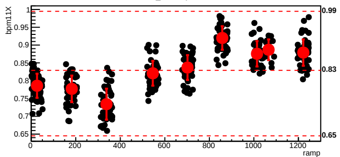
bmod_trim7,cyc=6041
