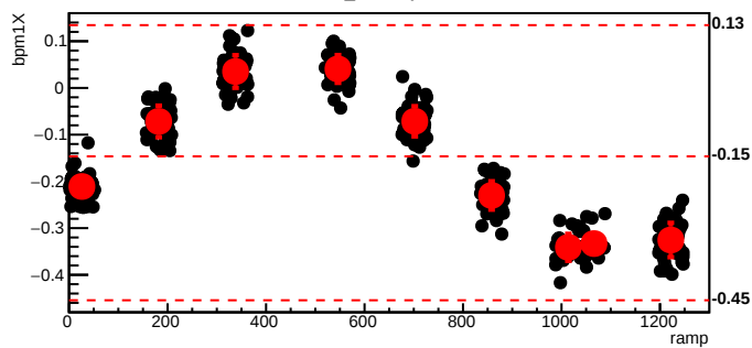
bmod_trim5,cyc=6041
