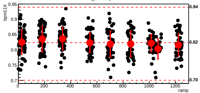
bmod_trim6,cyc=6041
