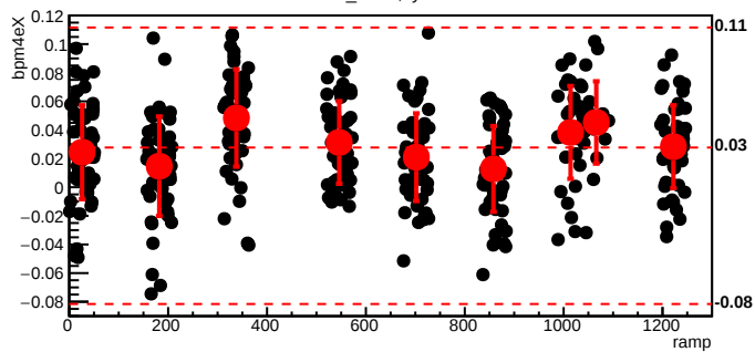
bmod_trim4,cyc=6041
