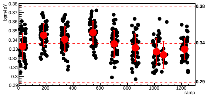
bmod_trim3,cyc=6041
