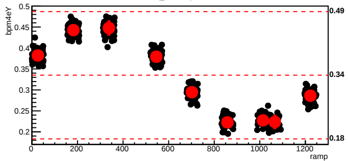
bmod_trim4,cyc=6041
