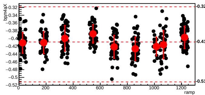
bmod_trim6,cyc=6050
