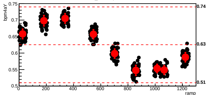
bmod_trim2,cyc=6050
