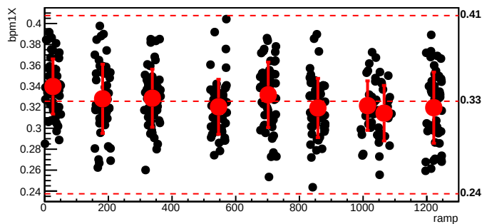
bmod_trim2,cyc=6050
