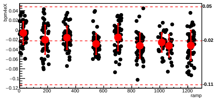
bmod_trim2,cyc=6050
