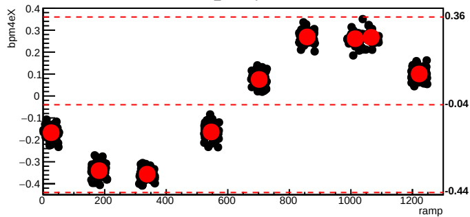
bmod_trim1,cyc=6050
