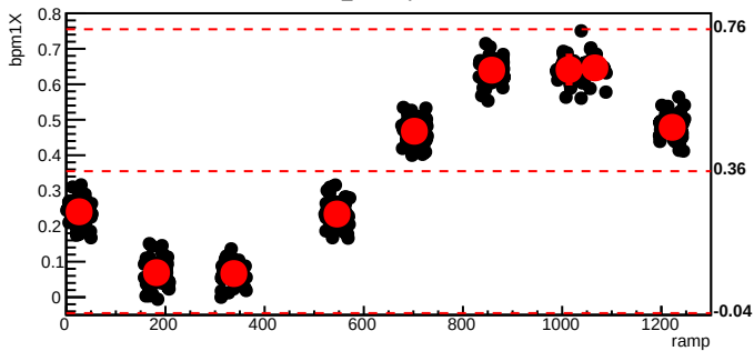
bmod_trim1,cyc=6050
