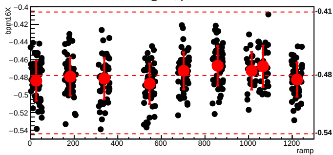
bmod_trim7,cyc=6050
