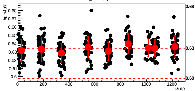
bmod_trim7,cyc=6050
