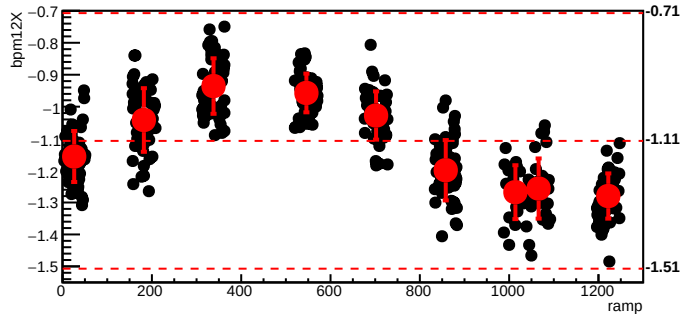
bmod_trim5,cyc=6050
