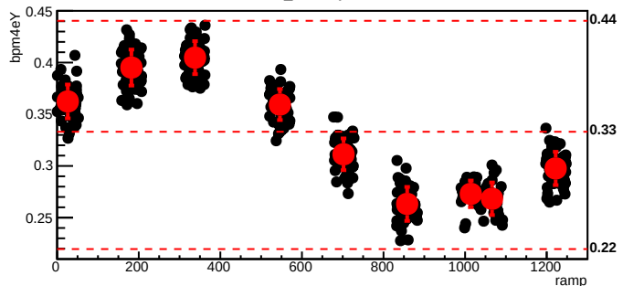
bmod_trim2,cyc=6050
