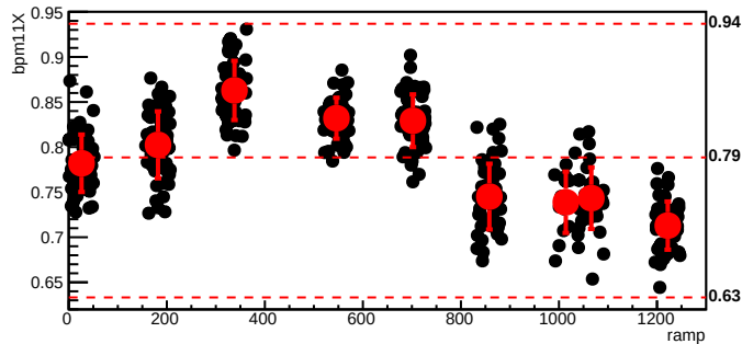
bmod_trim5,cyc=6050
