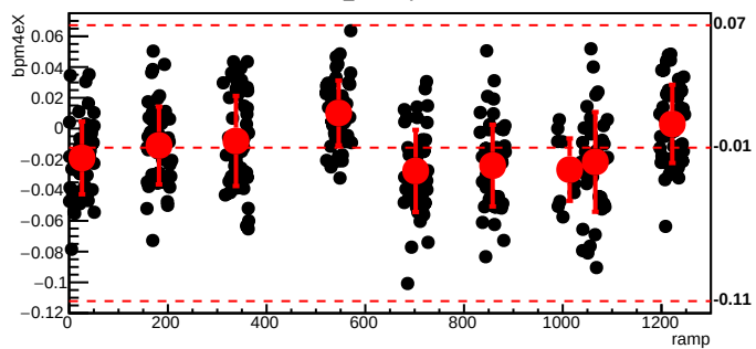
bmod_trim6,cyc=6050
