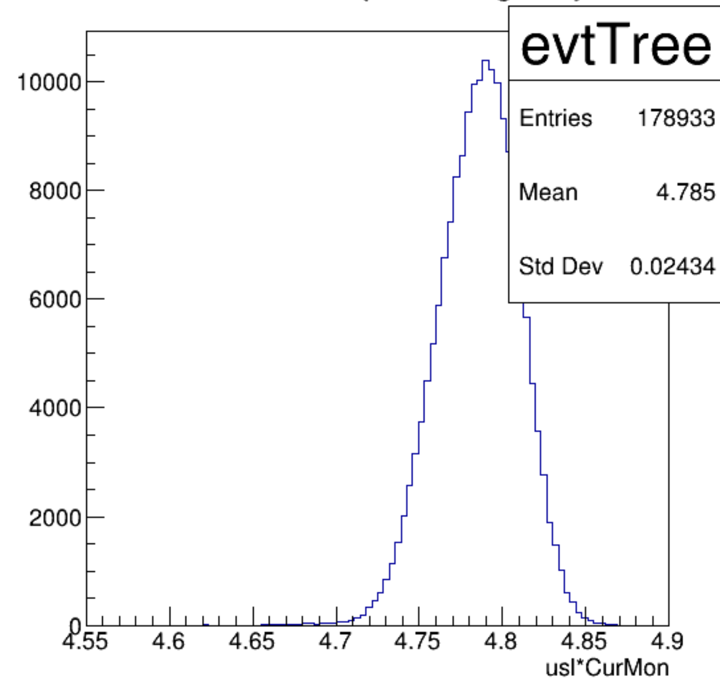
usl*CurMon {ErrorFlag==0}
