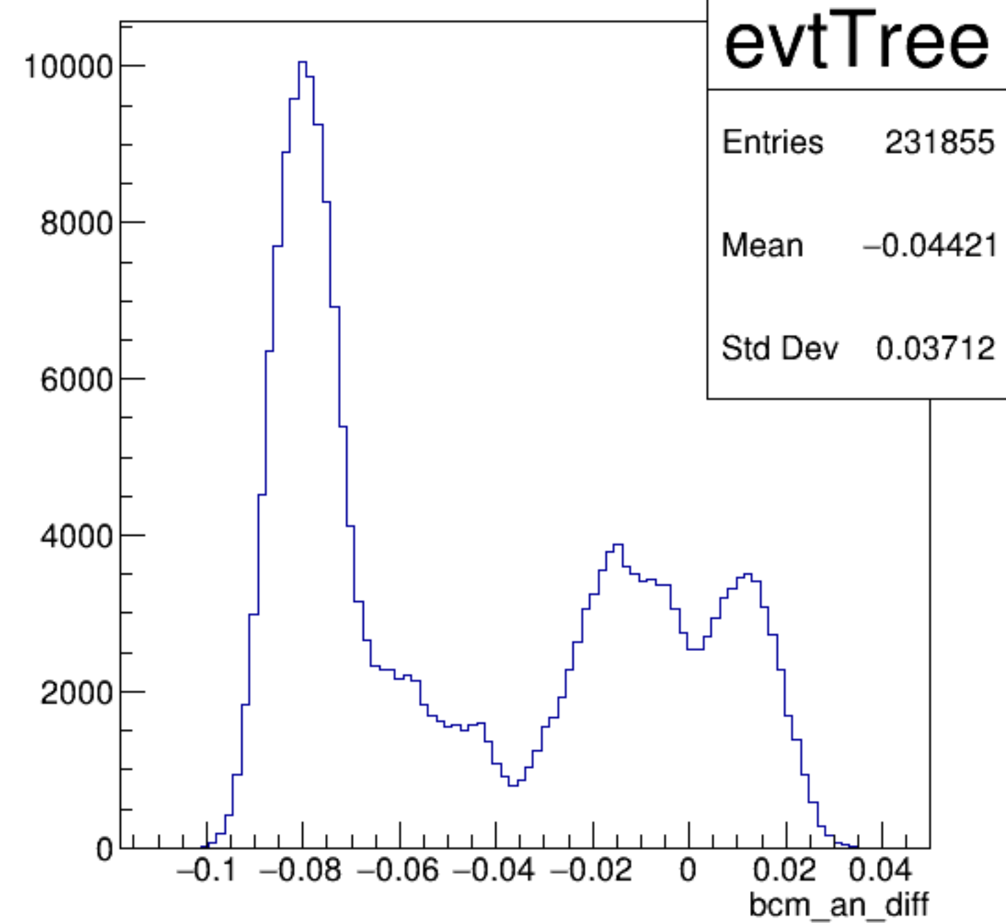
bcm_an_diff {ErrorFlag==0}
