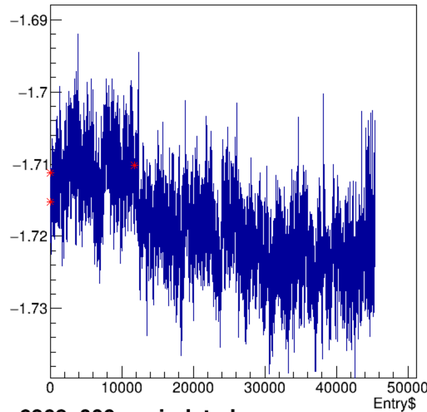
dsr*CurMon:Entry$
