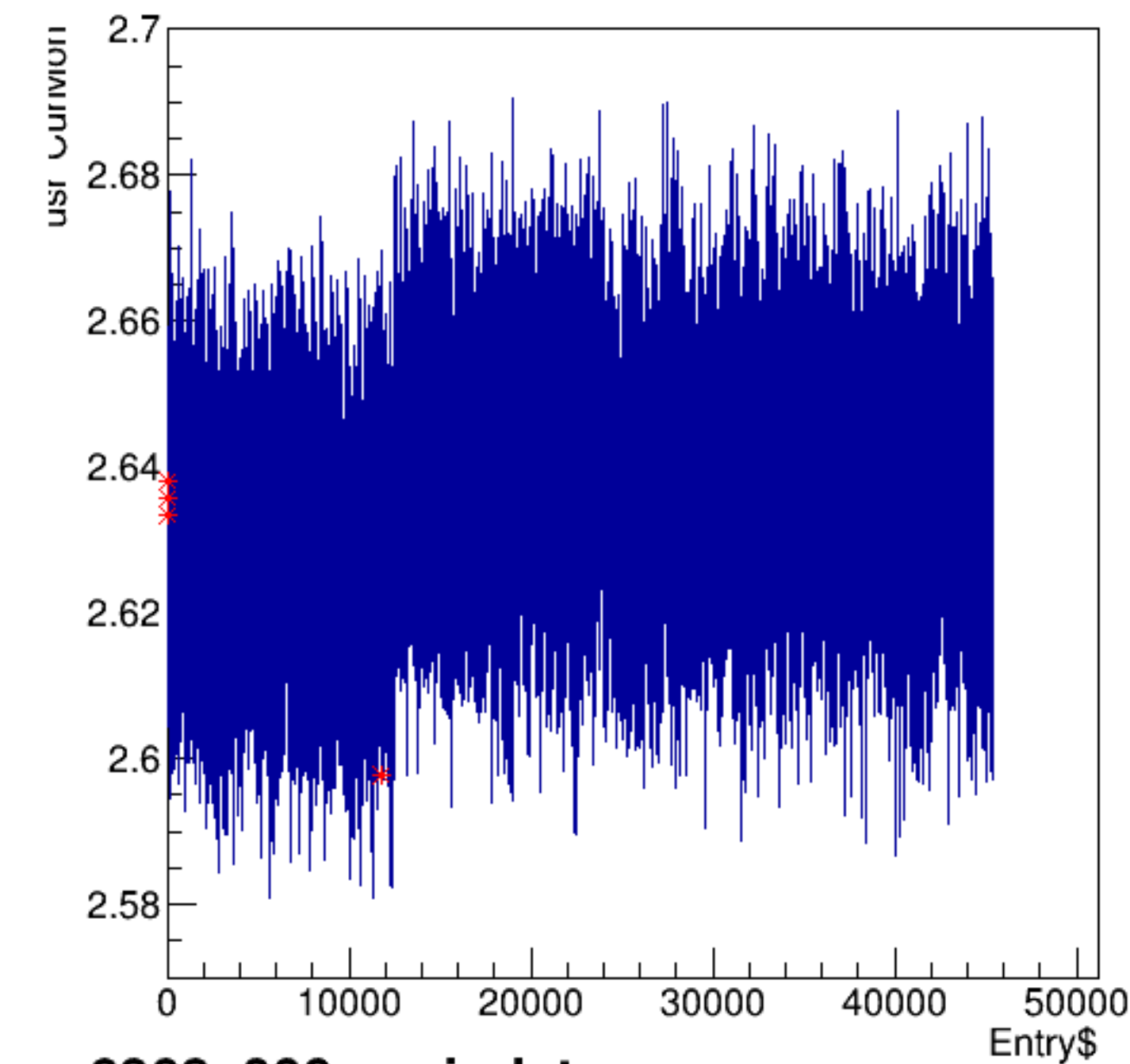
usr*CurMon:Entry$
