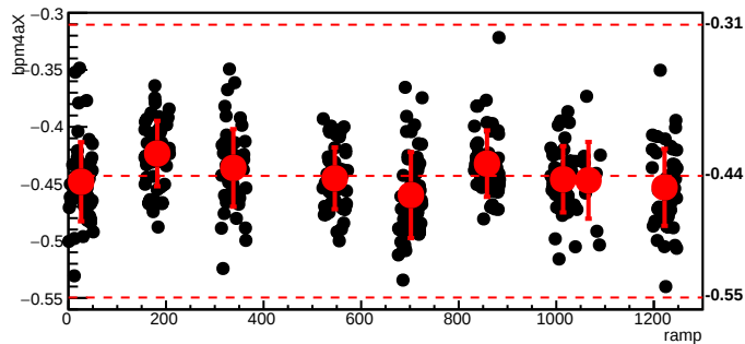
bmod_trim6,cyc=6093
