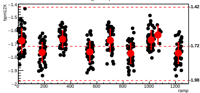
bmod_trim4,cyc=6093
