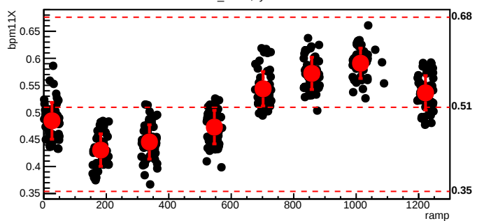
bmod_trim1,cyc=6093
