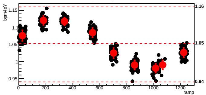
bmod_trim2,cyc=6093
