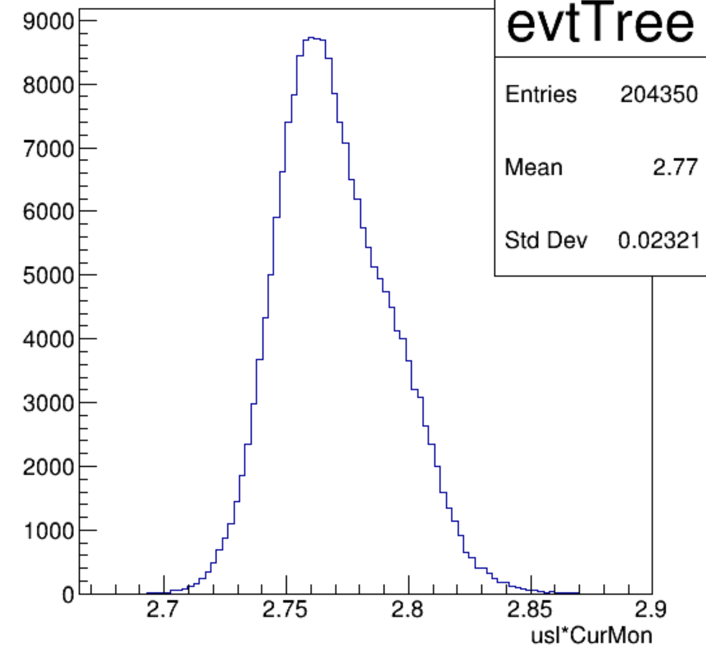
usl*CurMon {ErrorFlag==0}
