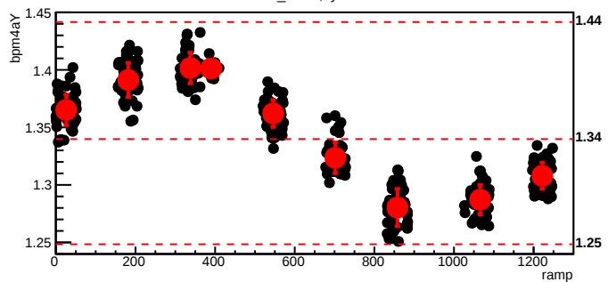
bmod_trim6,cyc=6072
