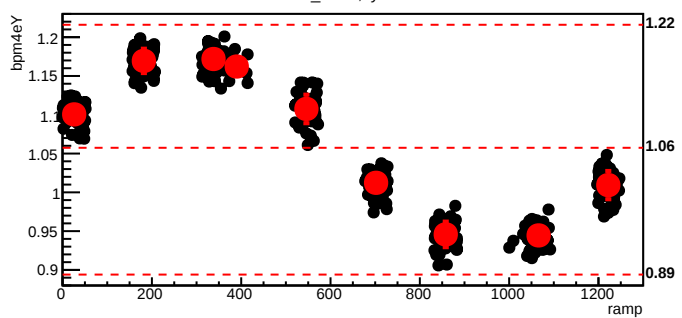
bmod_trim4,cyc=6072
