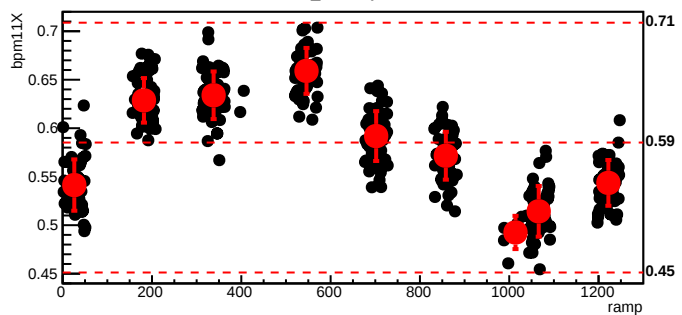
bmod_trim5,cyc=6072
