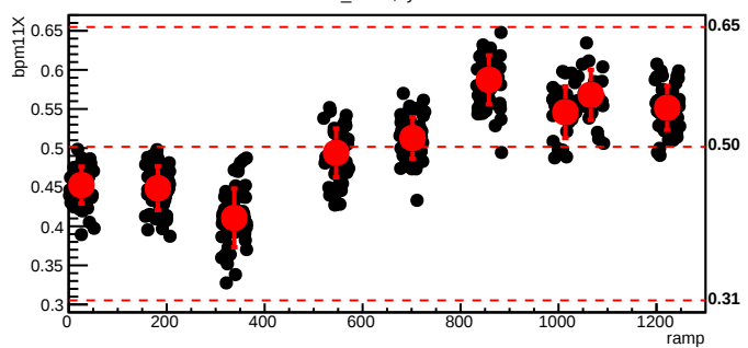
bmod_trim1,cyc=6074
