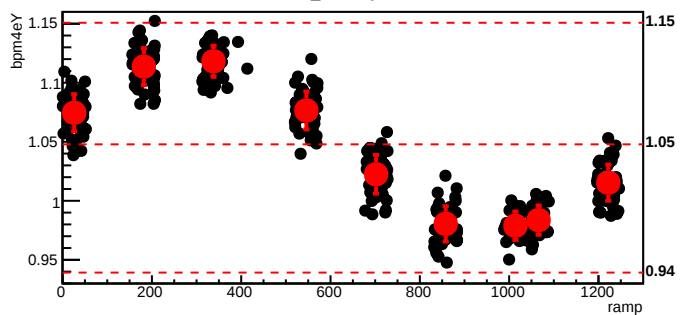
bmod_trim2,cyc=6074
