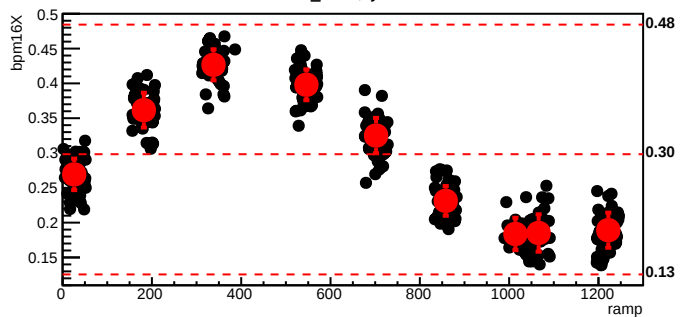
bmod_trim3,cyc=6074
