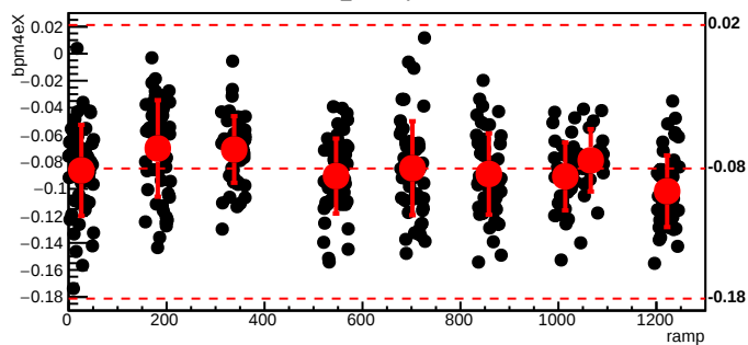
bmod_trim7,cyc=6074
