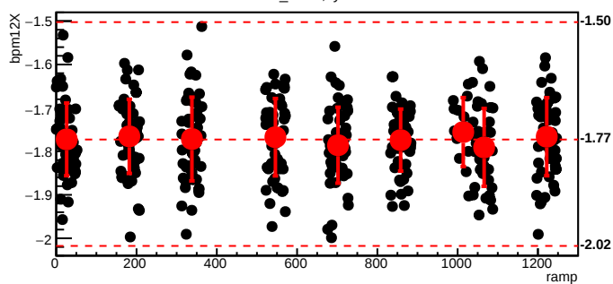
bmod_trim6,cyc=6078
