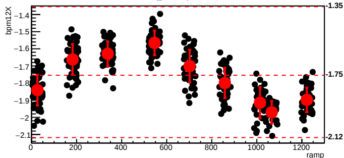
bmod_trim5,cyc=6078
