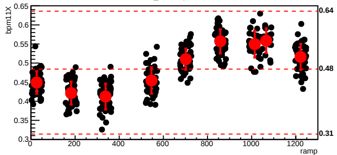
bmod_trim7,cyc=6078
