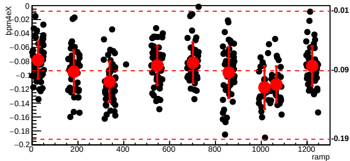
bmod_trim4,cyc=6078
