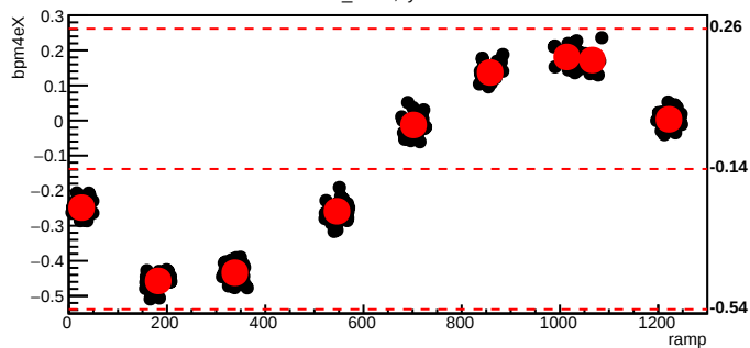
bmod_trim1,cyc=6075
