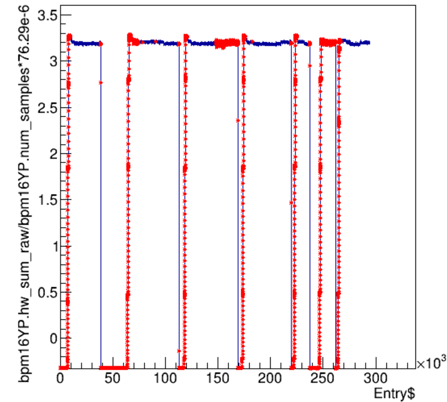
bpm16YP.hw_sum_raw/bpm16YP.num_samples*76.29e-6:Entry$
