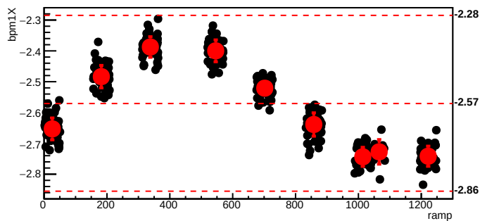
bmod_trim5,cyc=6080
