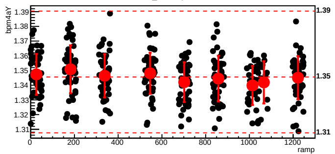
bmod_trim1,cyc=6080
