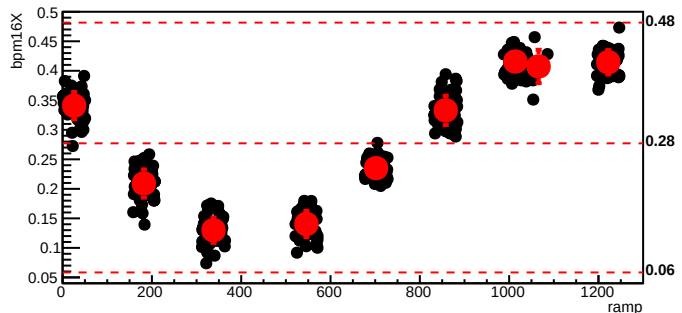
bmod_trim5,cyc=6080
