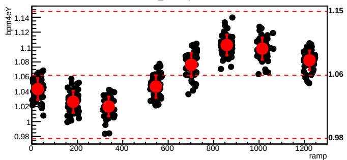
bmod_trim6,cyc=6080
