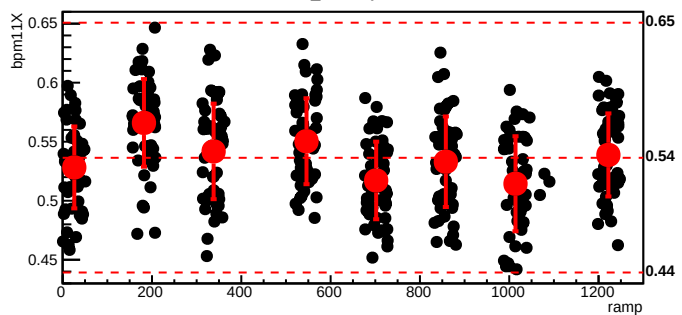
bmod_trim6,cyc=6082
