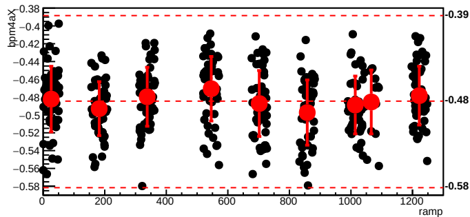
bmod_trim2,cyc=6082
