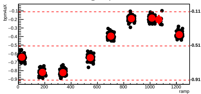
bmod_trim1,cyc=6082
