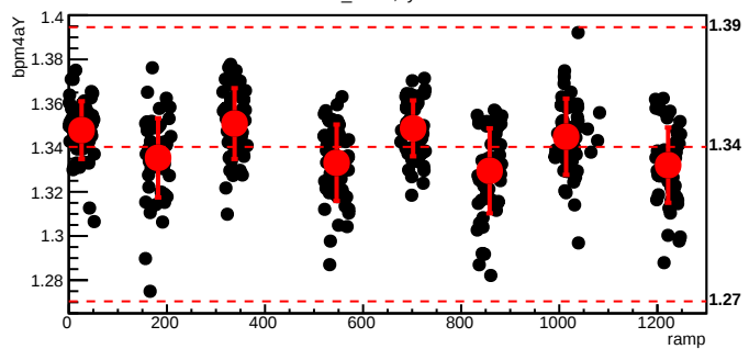
bmod_trim1,cyc=6083
