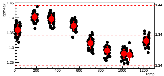
bmod_trim6,cyc=6083
