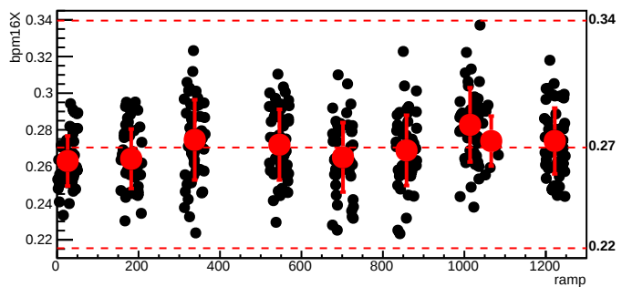
bmod_trim4,cyc=6083
