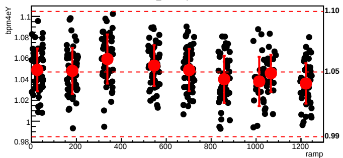
bmod_trim3,cyc=6083
