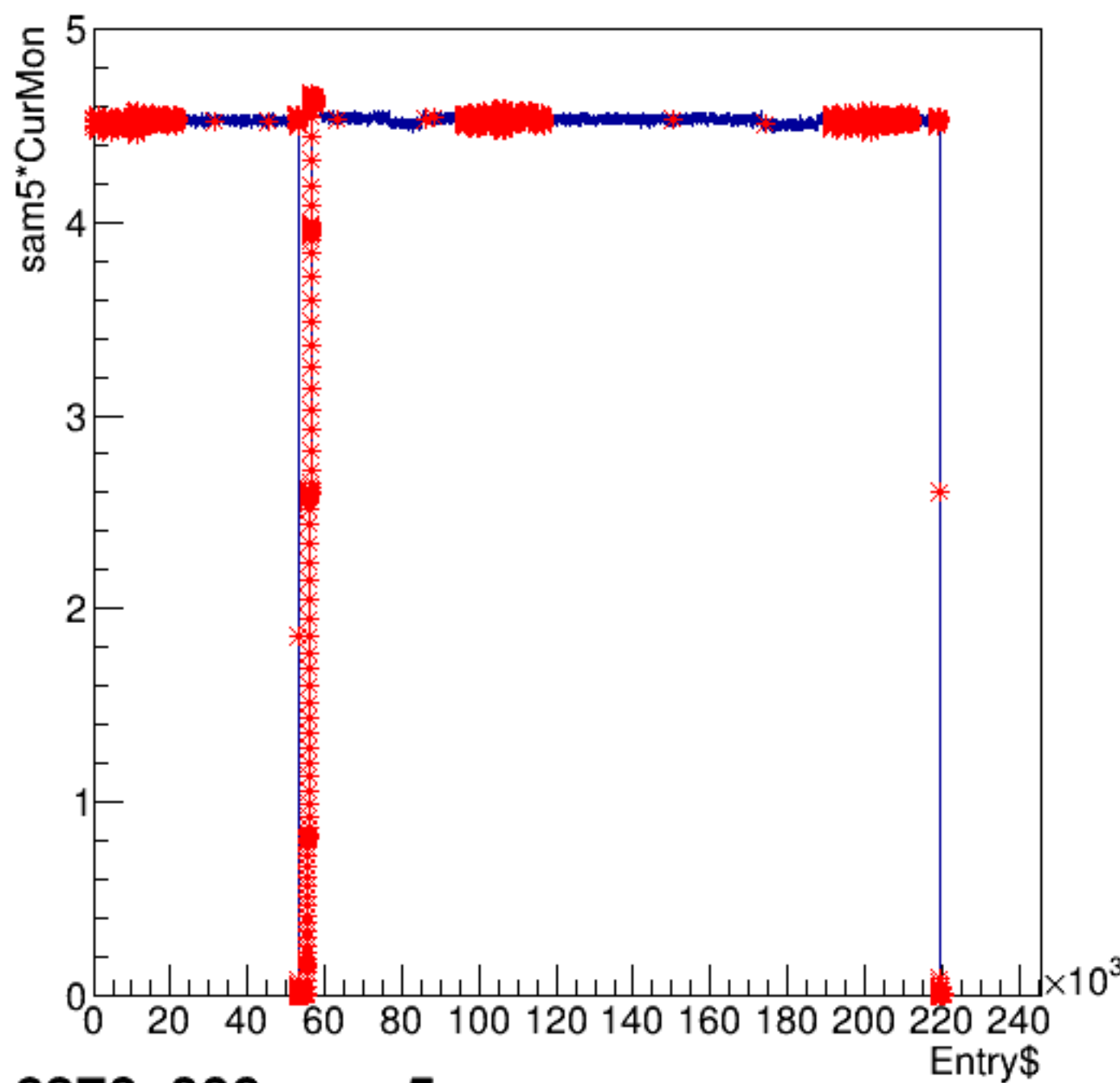
sam5*CurMon:Entry$
