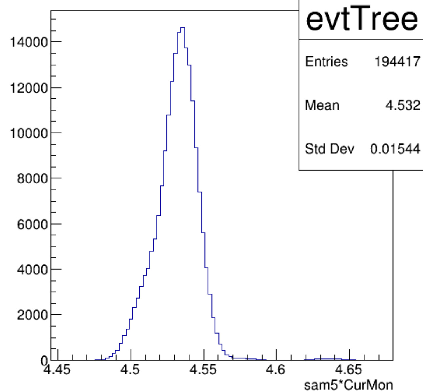
sam5*CurMon {ErrorFlag==0}
