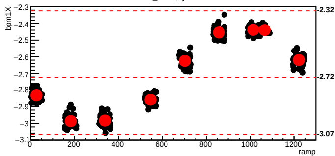
bmod_trim1,cyc=6087
