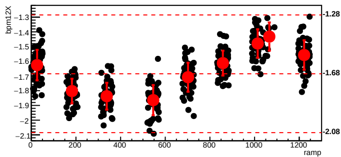
bmod_trim3,cyc=6087
