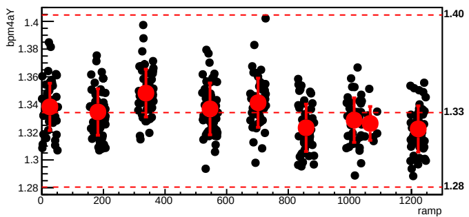
bmod_trim3,cyc=6087
