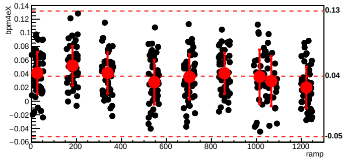
bmod_trim6,cyc=6095
