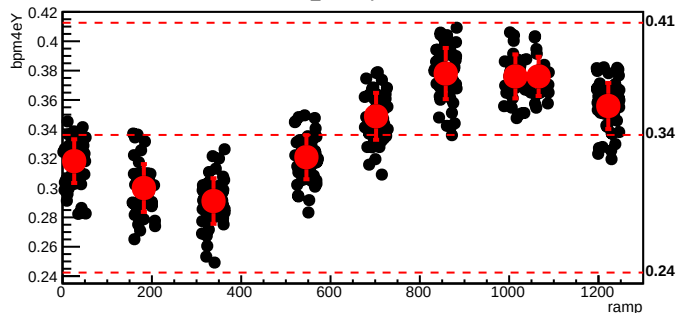
bmod_trim6,cyc=6095
