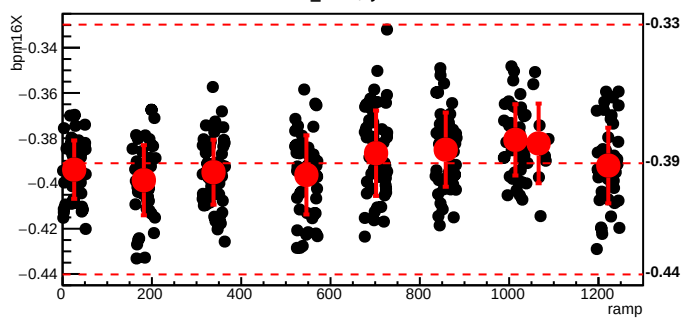
bmod_trim7,cyc=6095
