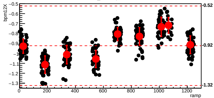
bmod_trim1,cyc=6095
