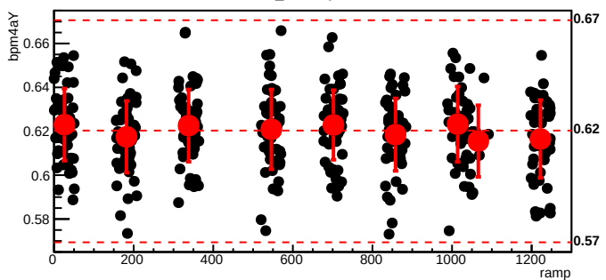
bmod_trim1,cyc=6095
