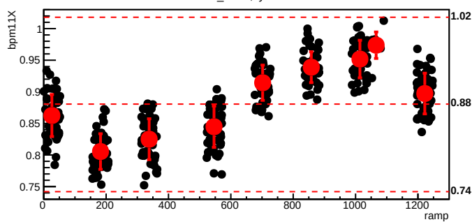
bmod_trim7,cyc=6095
