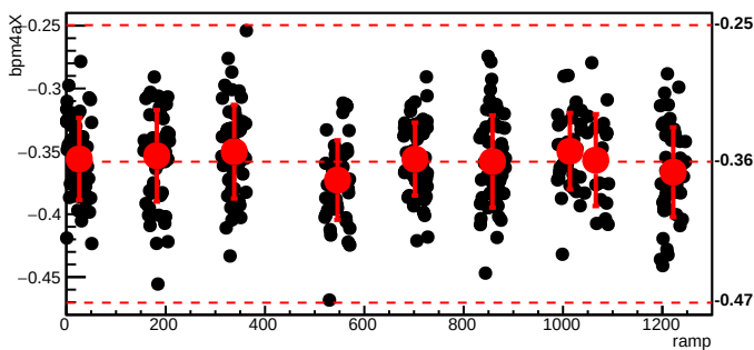
bmod_trim4,cyc=6095
