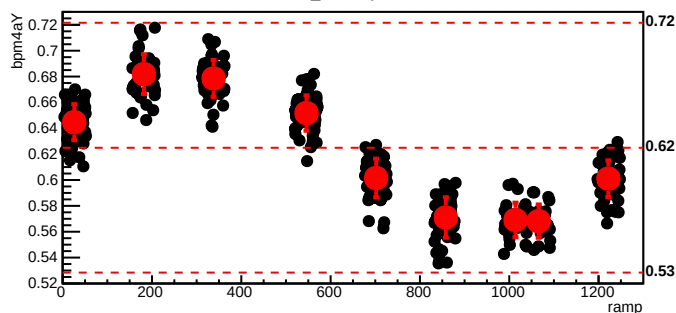
bmod_trim6,cyc=6095
