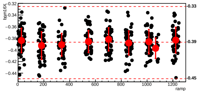
bmod_trim2,cyc=6095
