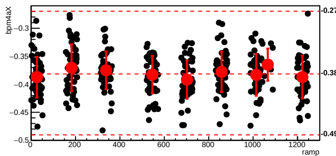
bmod_trim2,cyc=6095
