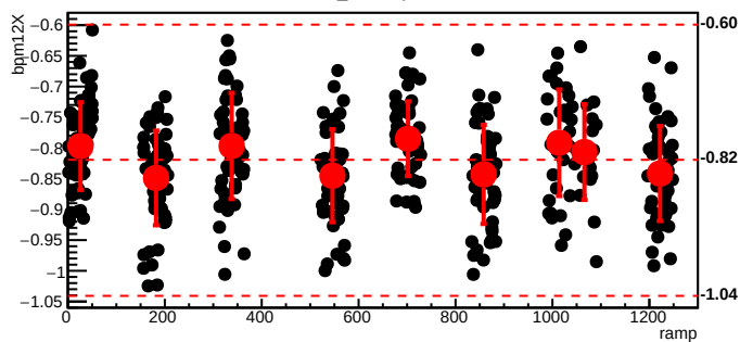
bmod_trim4,cyc=6095
