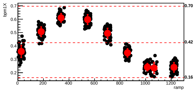
bmod_trim5,cyc=6095
