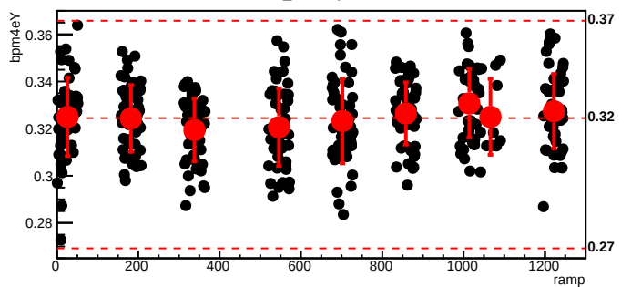
bmod_trim5,cyc=6098
