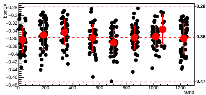
bmod_trim2,cyc=6098
