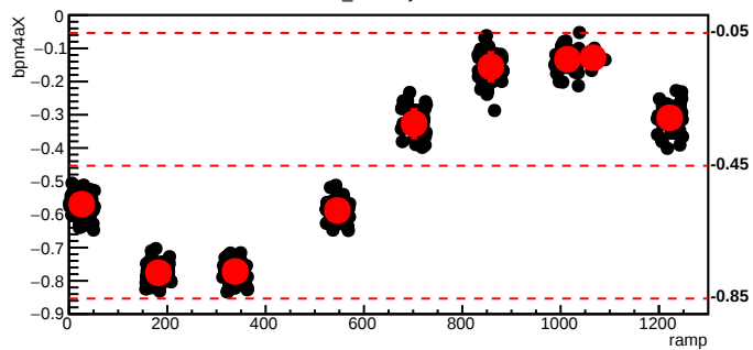
bmod_trim1,cyc=6098
