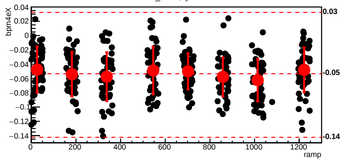
bmod_trim4,cyc=6098
