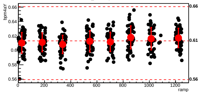
bmod_trim7,cyc=6098
