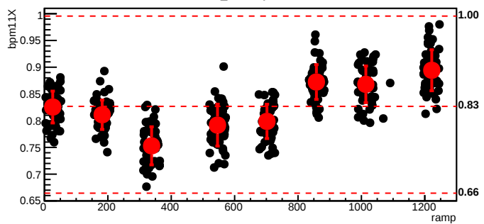
bmod_trim3,cyc=6098
