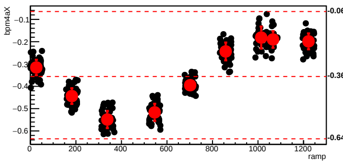
bmod_trim3,cyc=6099
