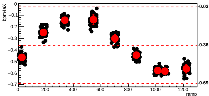
bmod_trim5,cyc=6099
