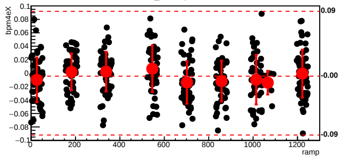
bmod_trim2,cyc=6099
