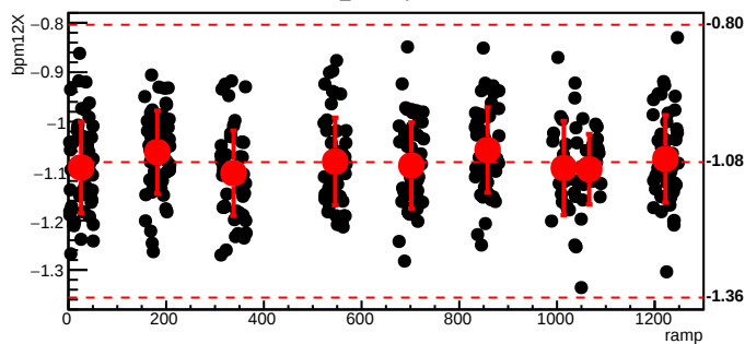
bmod_trim4,cyc=6099
