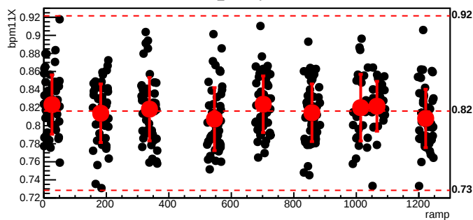
bmod_trim4,cyc=6099
