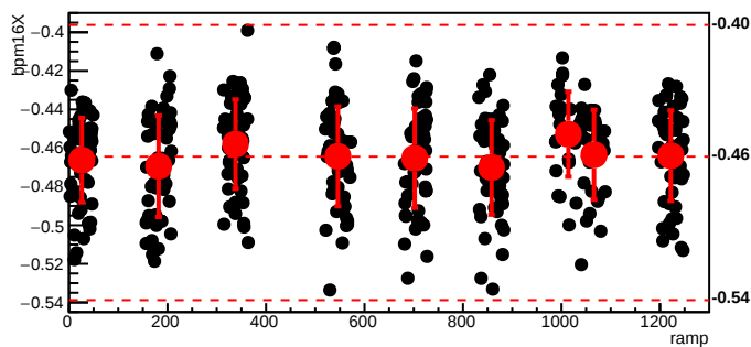
bmod_trim6,cyc=6099
