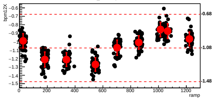
bmod_trim3,cyc=6099
