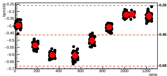
bmod_trim5,cyc=6099
