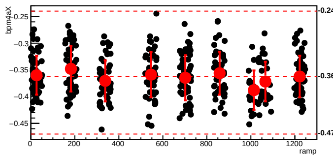
bmod_trim6,cyc=6099
