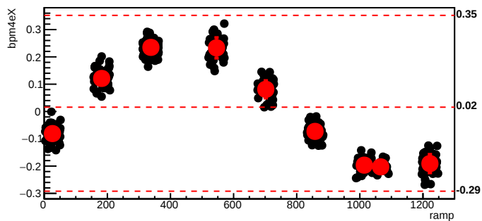
bmod_trim5,cyc=6099
