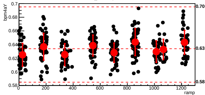
bmod_trim7,cyc=6099
