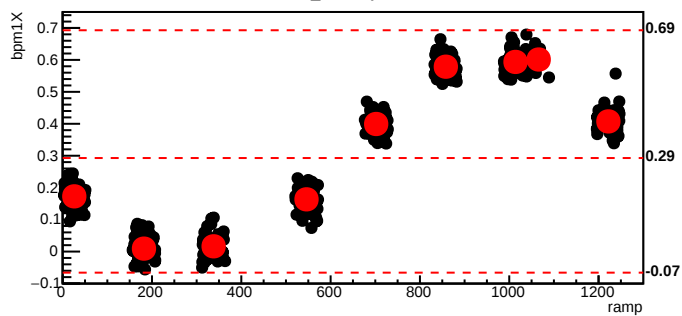
bmod_trim1,cyc=6099
