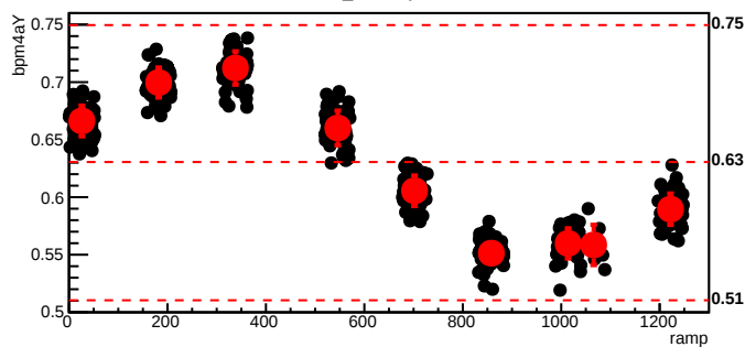
bmod_trim2,cyc=6099
