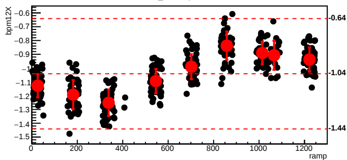
bmod_trim7,cyc=6099
