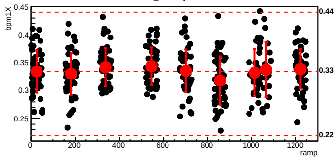
bmod_trim2,cyc=6103
