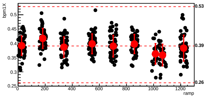
bmod_trim7,cyc=6103
