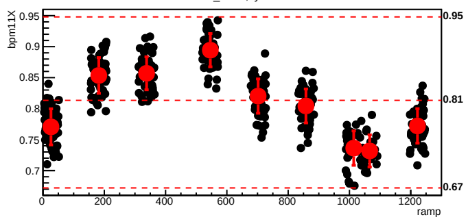
bmod_trim5,cyc=6103
