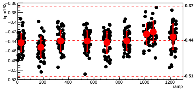
bmod_trim7,cyc=6103
