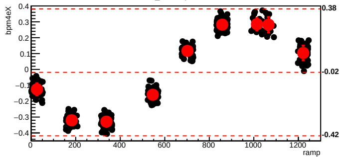
bmod_trim1,cyc=6103
