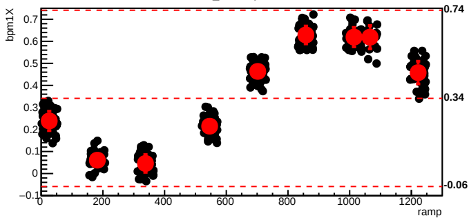
bmod_trim1,cyc=6103
