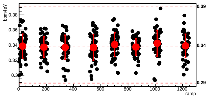
bmod_trim7,cyc=6114
