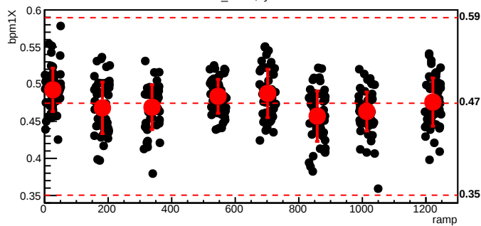
bmod_trim2,cyc=6114
