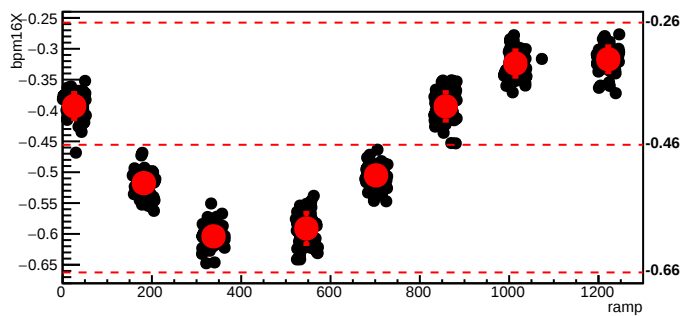
bmod_trim5,cyc=6114
