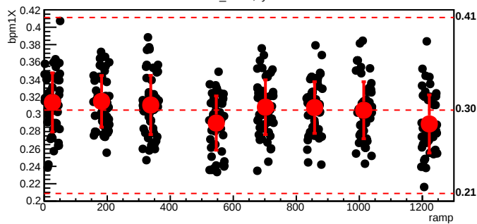
bmod_trim2,cyc=6113
