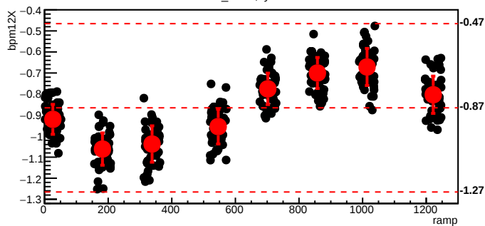
bmod_trim7,cyc=6113
