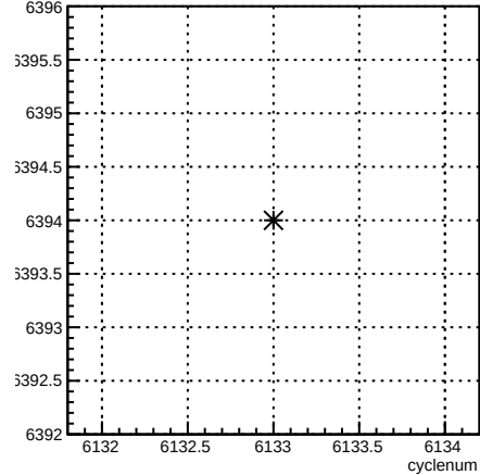
run:cyclenum {run == 6394}
