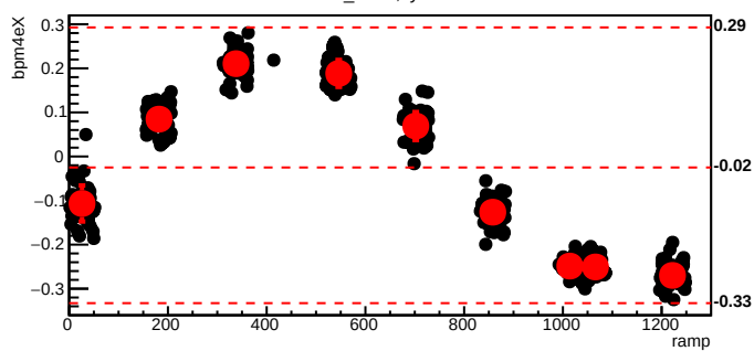
bmod_trim5,cyc=6134
