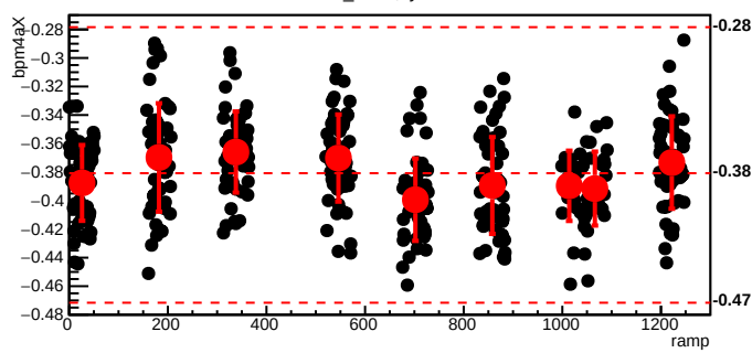
bmod_trim7,cyc=6134
