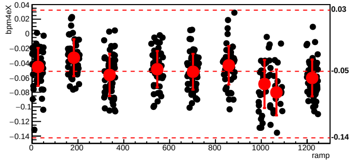
bmod_trim2,cyc=6134
