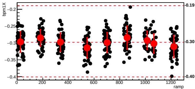
bmod_trim4,cyc=6134
