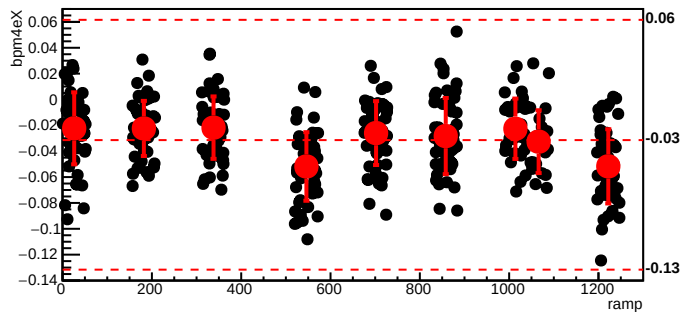
bmod_trim4,cyc=6134
