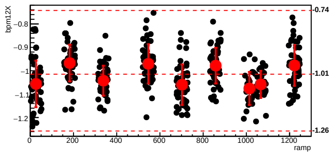
bmod_trim6,cyc=6134
