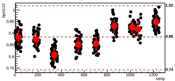
bmod_trim3,cyc=6134
