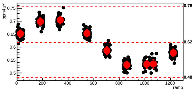
bmod_trim6,cyc=6134
