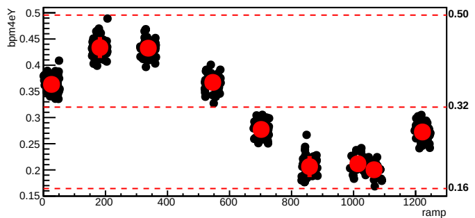
bmod_trim4,cyc=6134
