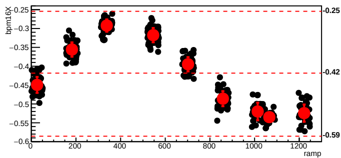
bmod_trim3,cyc=6134
