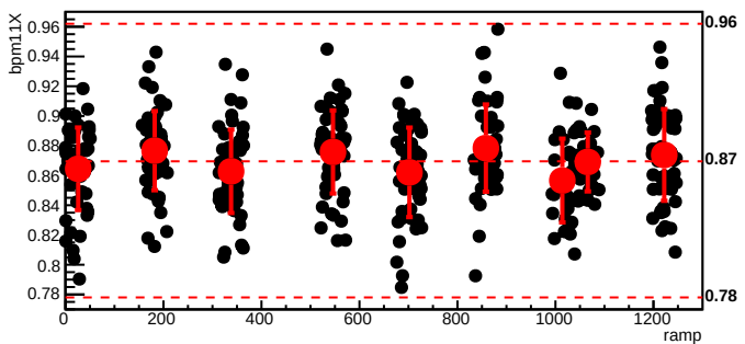
bmod_trim4,cyc=6134
