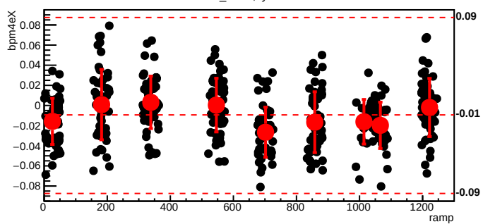
bmod_trim7,cyc=6134
