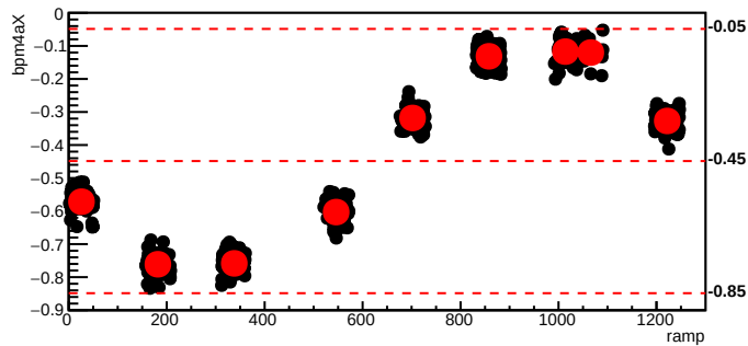
bmod_trim1,cyc=6134
