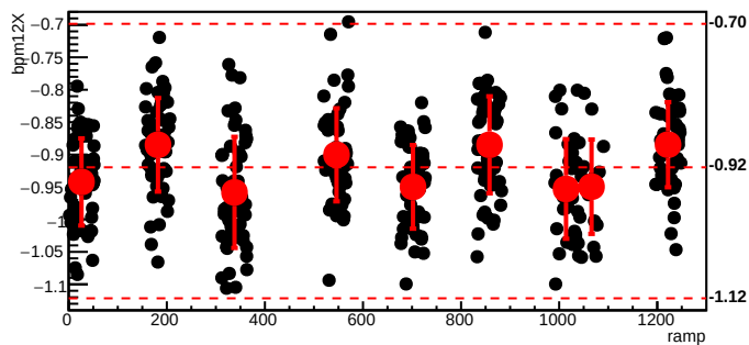
bmod_trim2,cyc=6134
