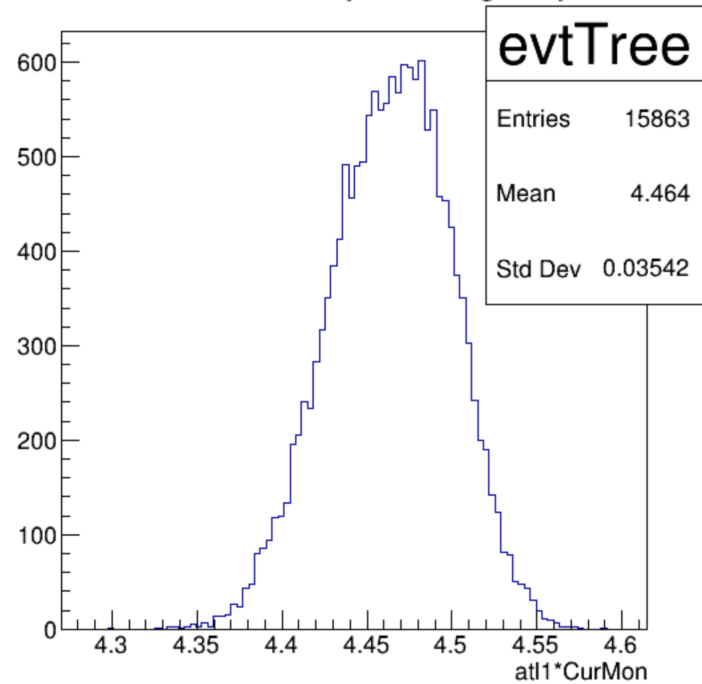
atl1*CurMon {ErrorFlag==0}
