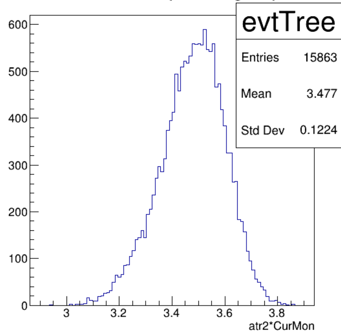
atr2*CurMon {ErrorFlag==0}
