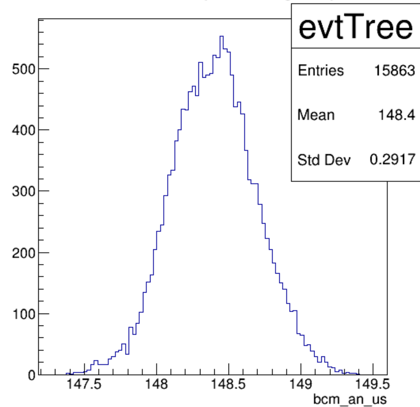
bcm_an_us {ErrorFlag==0}
