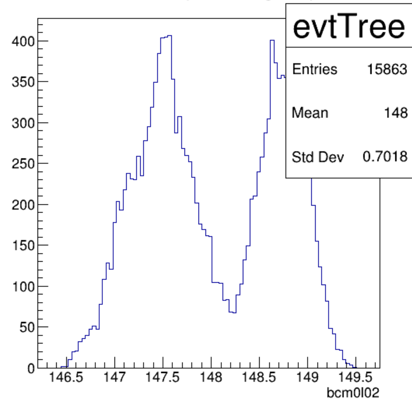
bcm0l02 {ErrorFlag==0}
