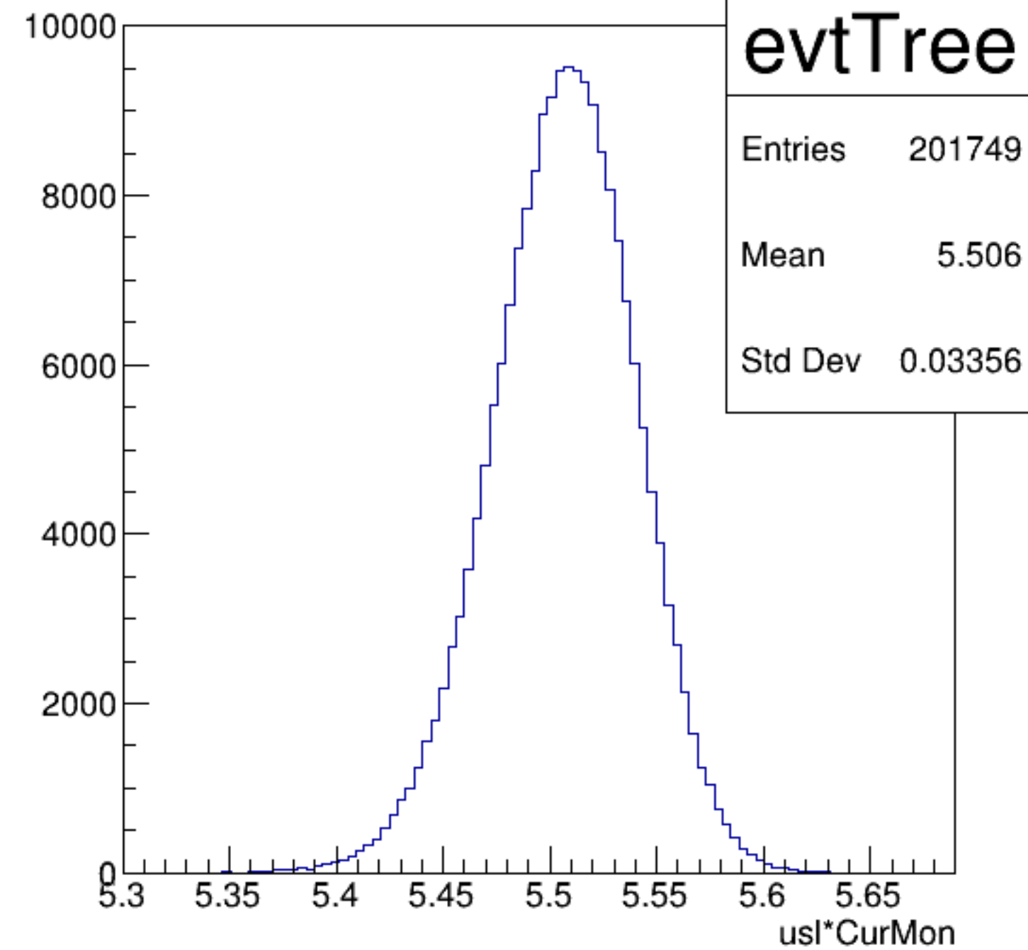
usl*CurMon {ErrorFlag==0}
