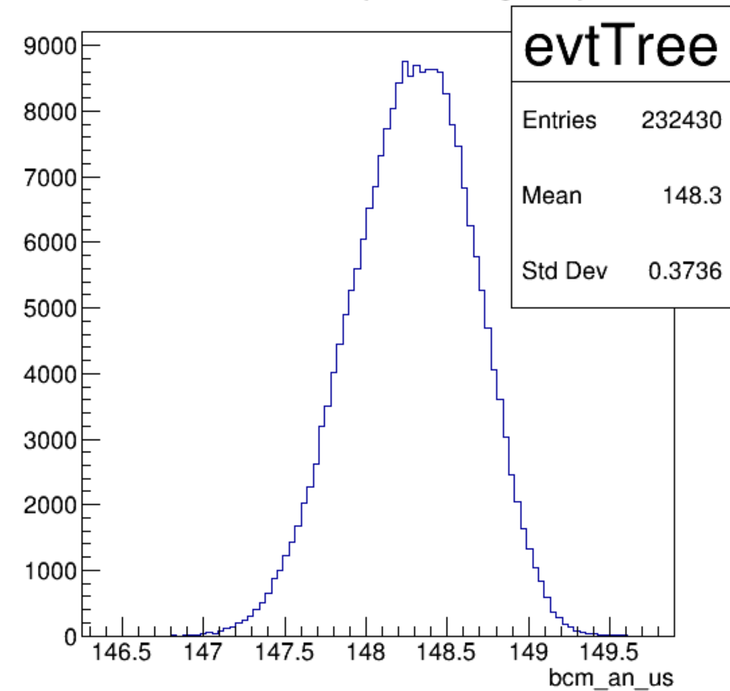
bcm_an_us {ErrorFlag==0}
