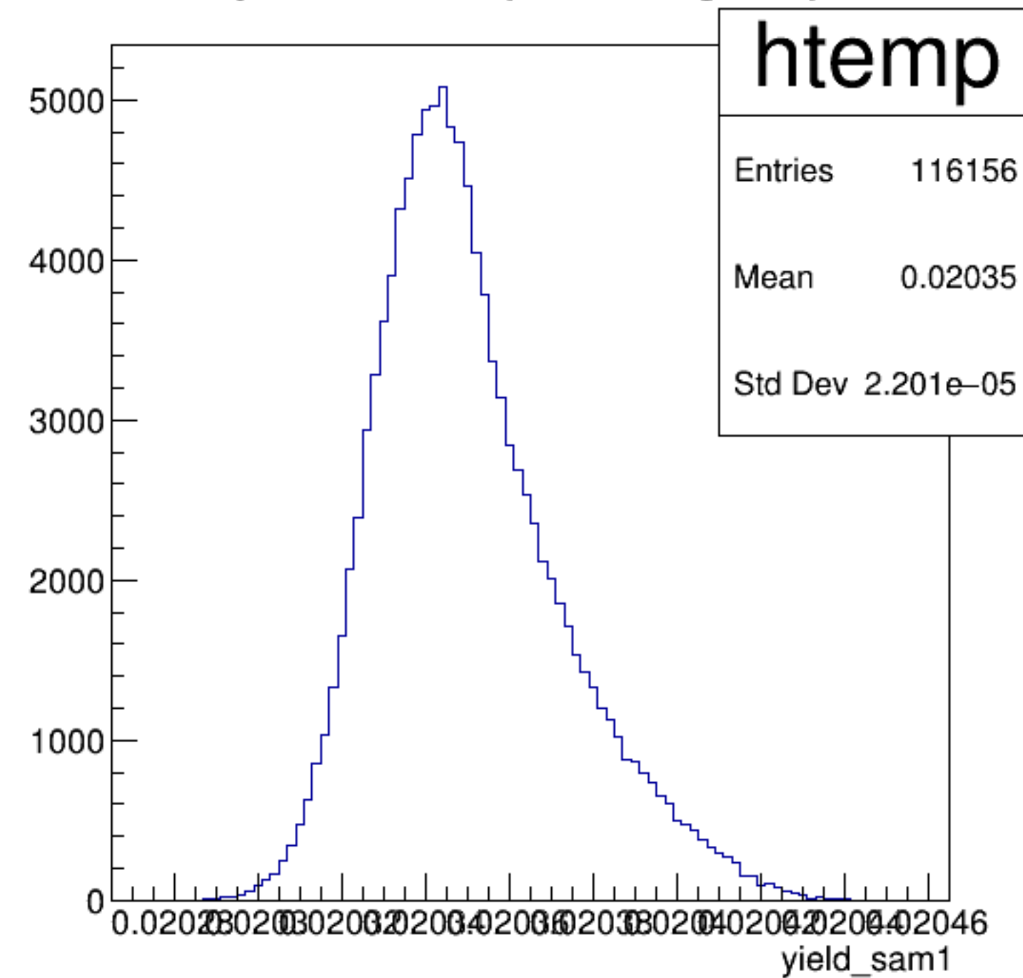
yield_sam1 {ErrorFlag==0}
