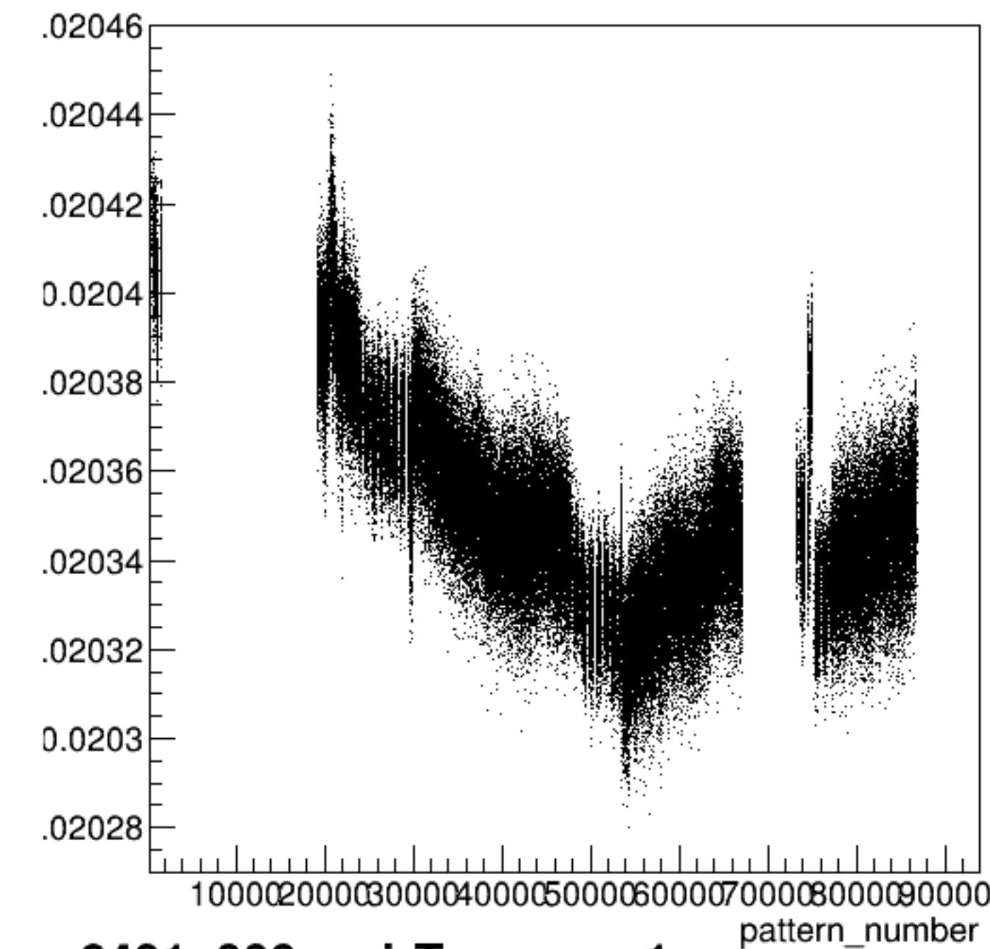
yield_sam1:pattern_number {ErrorFlag==0}
