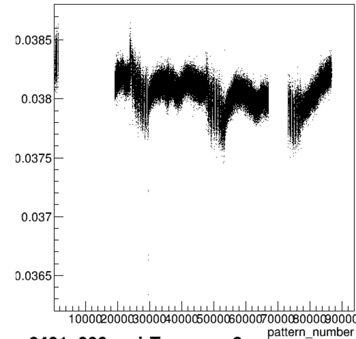
yield_sam3:pattern_number {ErrorFlag==0}
