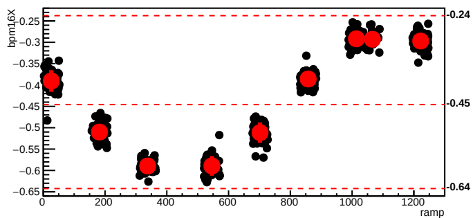
bmod_trim5,cyc=6156
