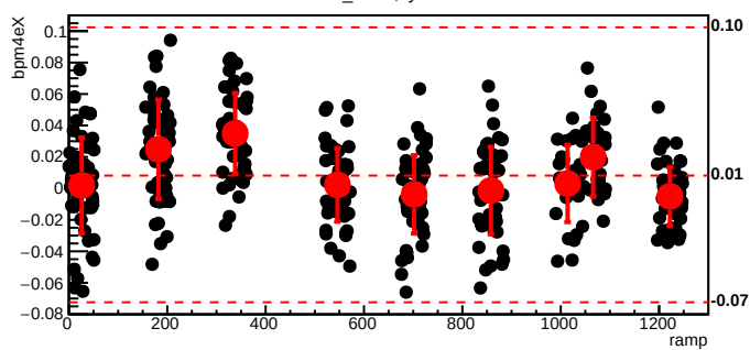
bmod_trim7,cyc=6156
