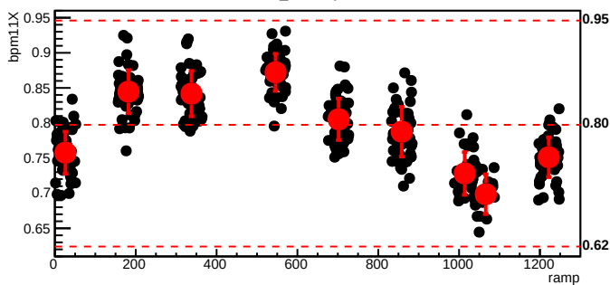
bmod_trim5,cyc=6156
