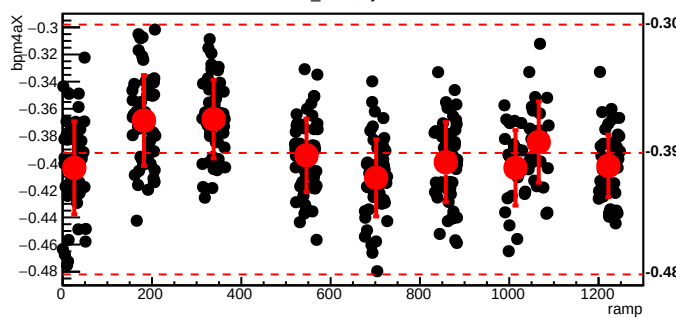
bmod_trim7,cyc=6156
