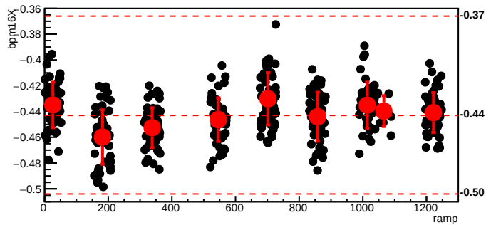
bmod_trim7,cyc=6157
