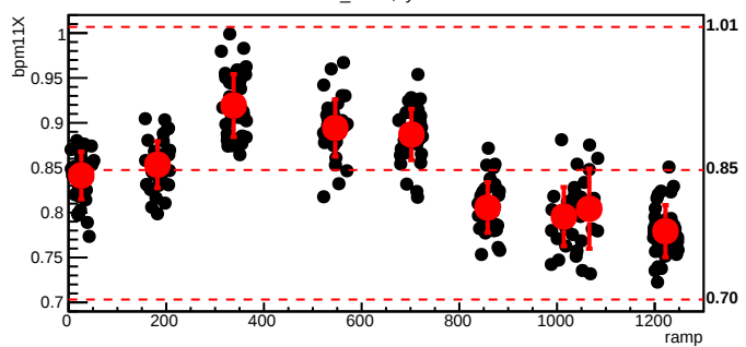
bmod_trim5,cyc=6157
