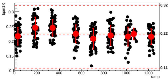
bmod_trim7,cyc=6157
