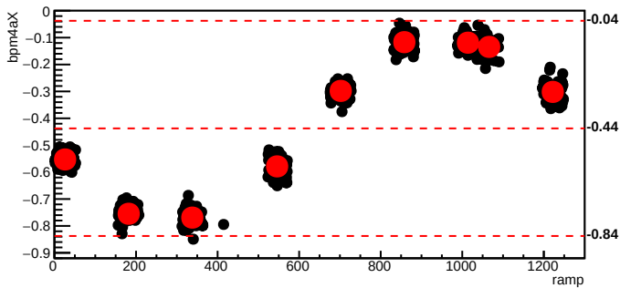
bmod_trim1,cyc=6164
