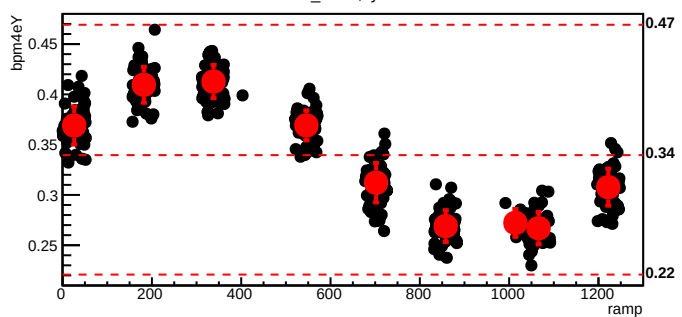
bmod_trim2,cyc=6164
