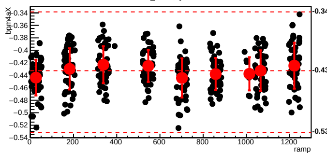
bmod_trim2,cyc=6164
