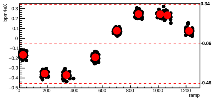
bmod_trim1,cyc=6164
