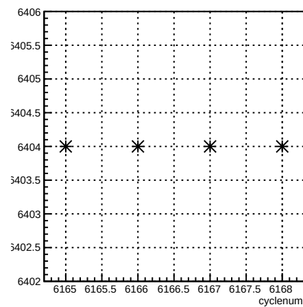
run:cyclenum {run == 6404}
