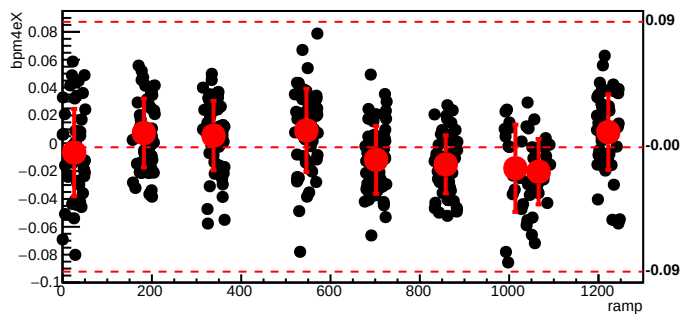
bmod_trim7,cyc=6170
