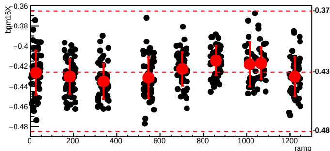
bmod_trim7,cyc=6170
