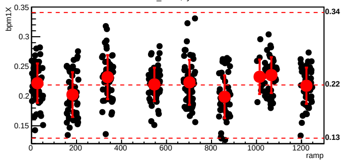
bmod_trim4,cyc=6170
