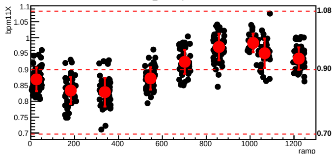
bmod_trim7,cyc=6170
