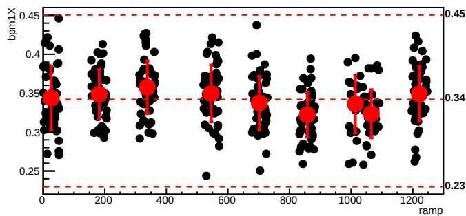
bmod_trim7,cyc=6170
