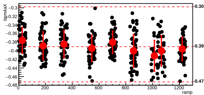
bmod_trim6,cyc=6170
