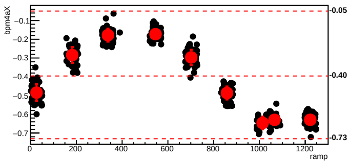
bmod_trim5,cyc=6170
