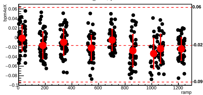
bmod_trim6,cyc=6170
