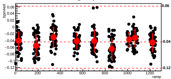
bmod_trim4,cyc=6170
