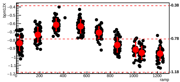
bmod_trim5,cyc=6170
