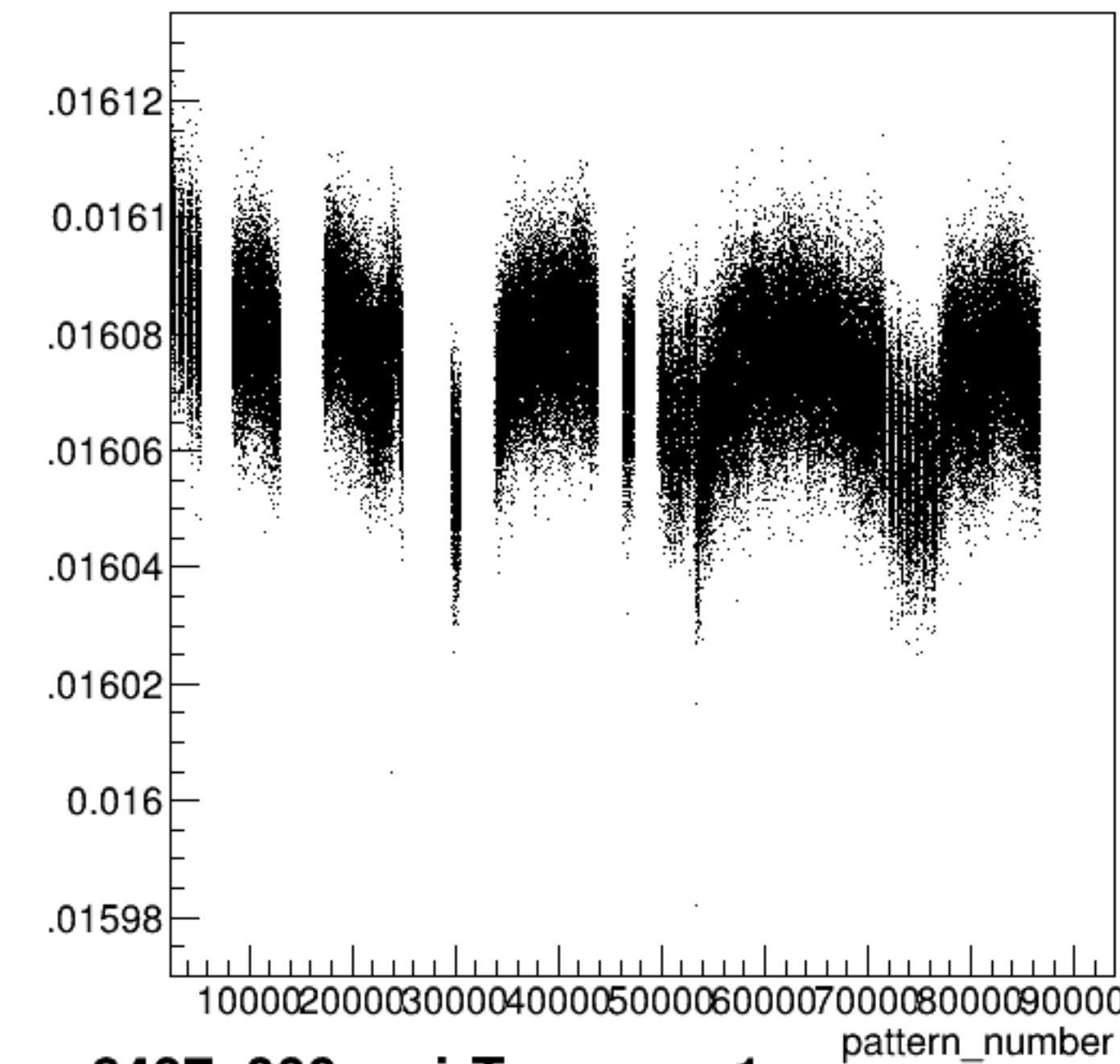
yield_sam1:pattern_number {ErrorFlag==0}
