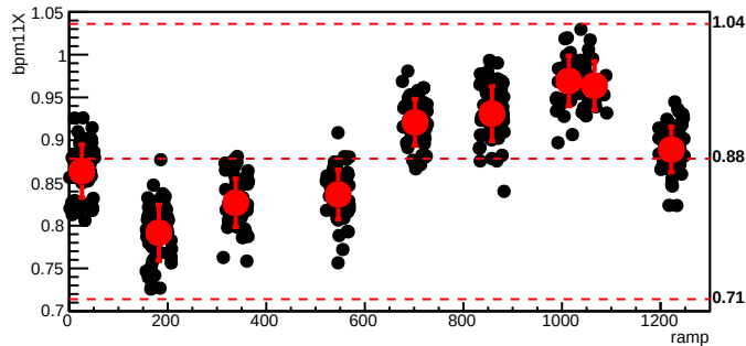
bmod_trim7,cyc=6178
