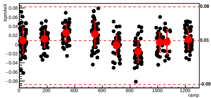
bmod_trim7,cyc=6178
