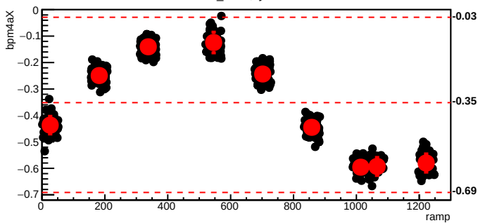
bmod_trim5,cyc=6178
