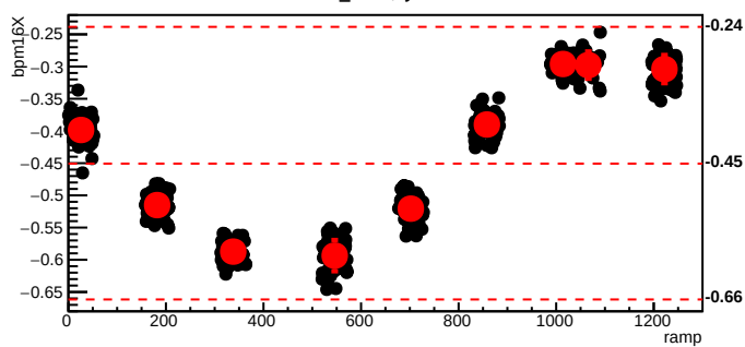
bmod_trim5,cyc=6178
