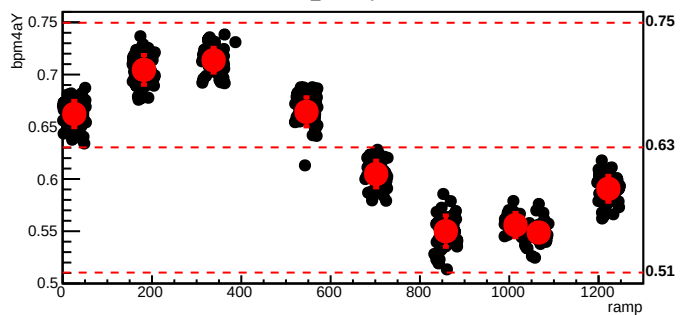
bmod_trim2,cyc=6178
