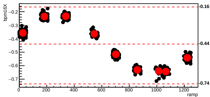
bmod_trim1,cyc=6178
