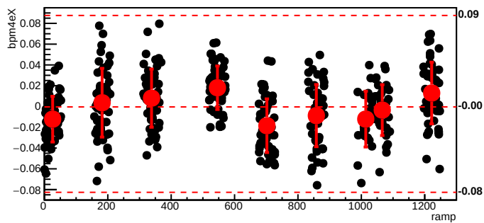
bmod_trim2,cyc=6178
