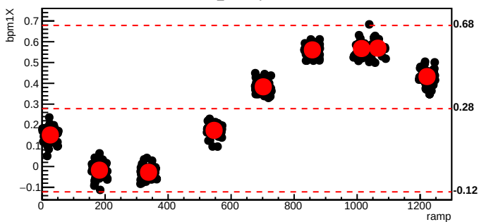
bmod_trim1,cyc=6178
