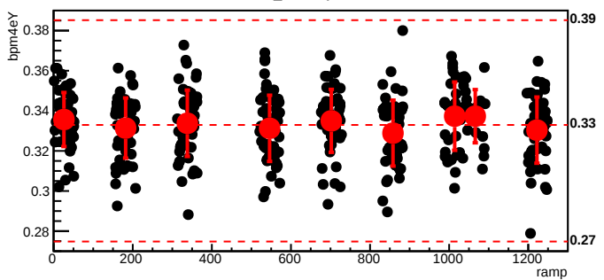
bmod_trim1,cyc=6176
