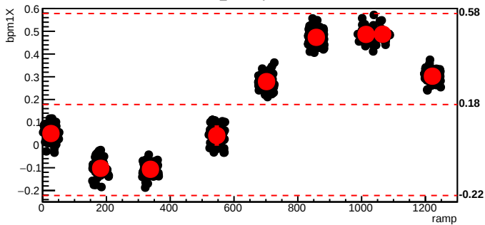
bmod_trim1,cyc=6176
