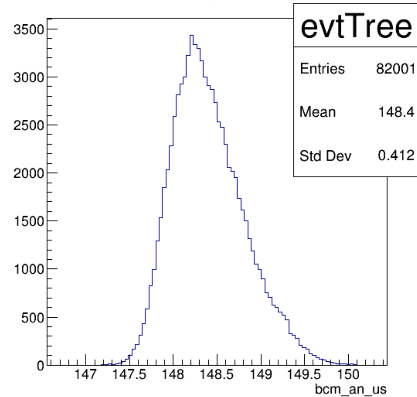
bcm_an_us {ErrorFlag==0}
