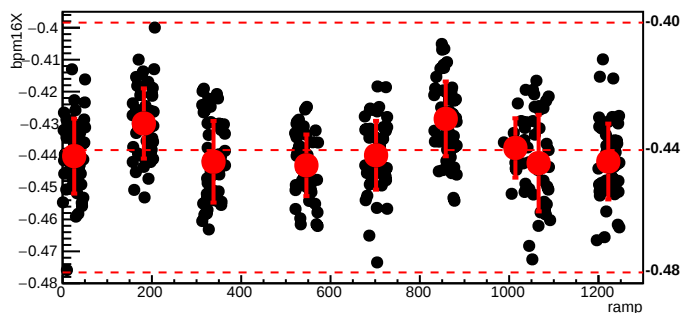
bmod_trim7,cyc=6179
