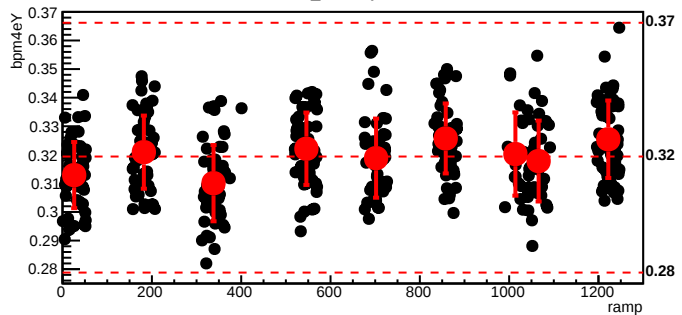
bmod_trim5,cyc=6179
