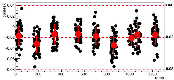
bmod_trim7,cyc=6179
