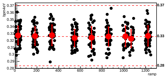
bmod_trim1,cyc=6179
