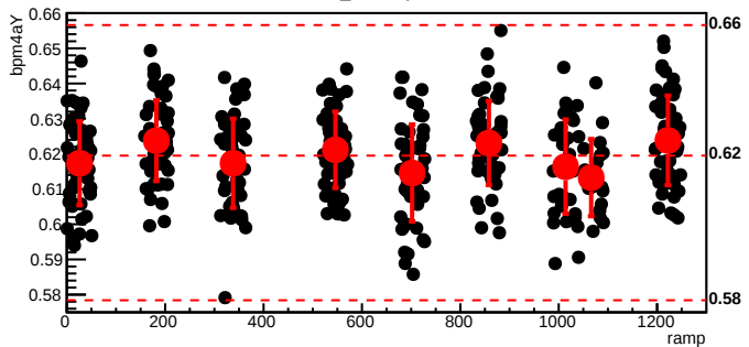
bmod_trim1,cyc=6179
