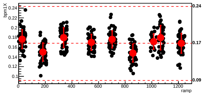
bmod_trim7,cyc=6179
