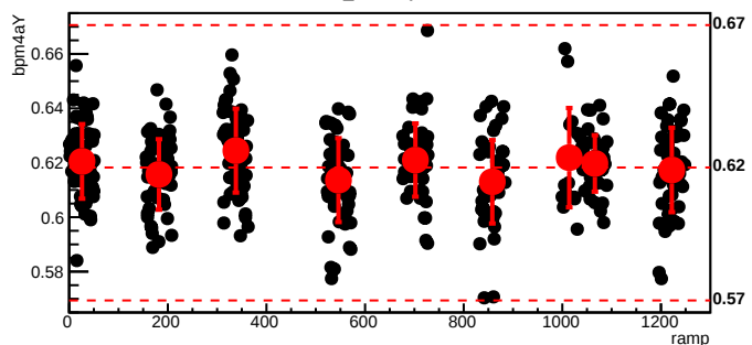
bmod_trim7,cyc=6179
