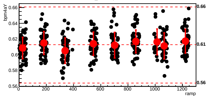
bmod_trim5,cyc=6179
