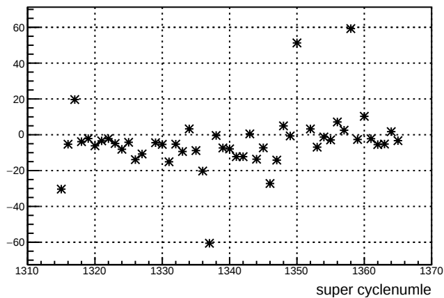
dsr_4aY : slug 27
