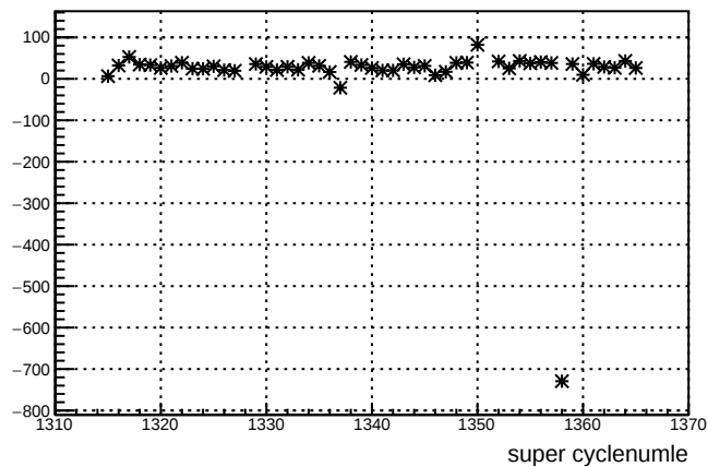
usl_4aY : slug 27
