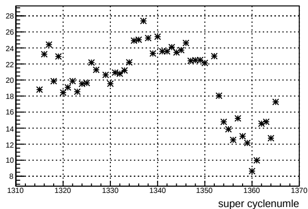
usr_4eY : slug 27
