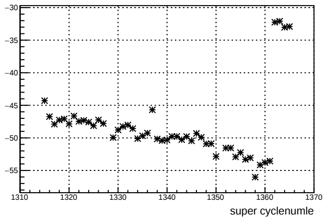
dsr_11X12X : slug 27
