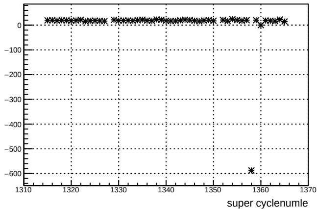
dd_us_4ay
