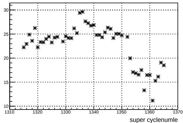
usl_4eY : slug 27
