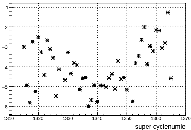
dsr_11X12X : slug 27
