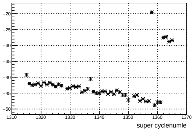
usl_11X12X : slug 27
