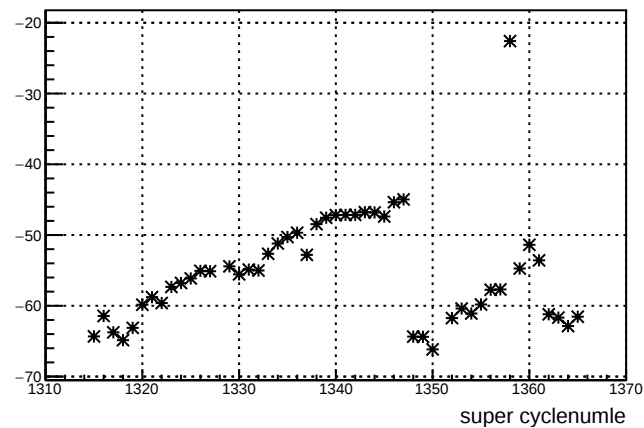
usl_4eY : slug 27
