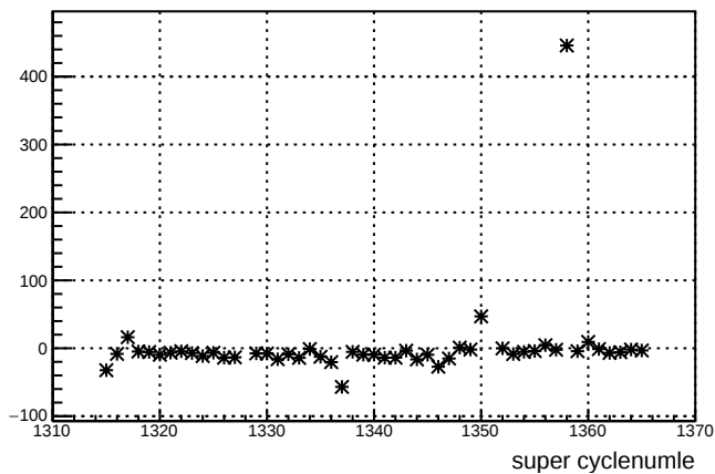
usr_4aY : slug 27
