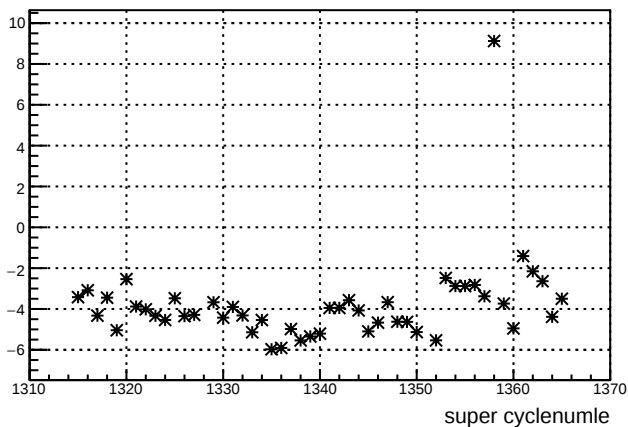
usl_11X12X : slug 27
