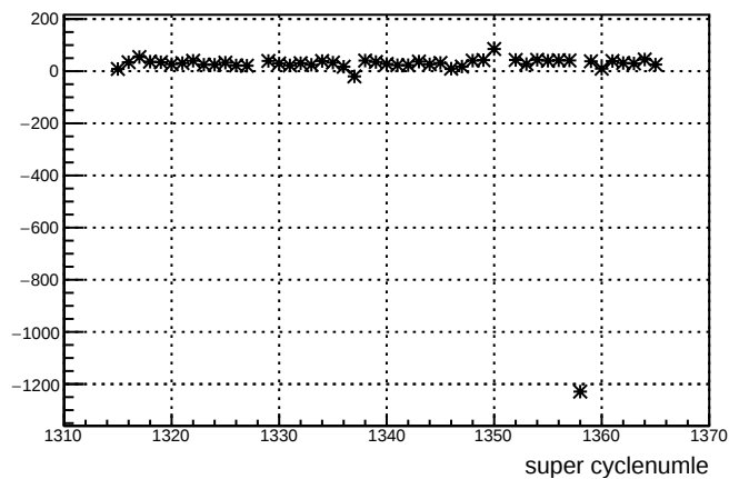
dsl_4aY
