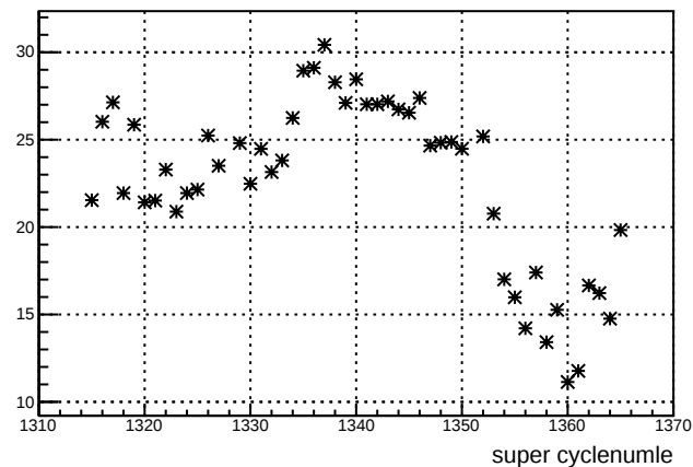
dsr_4eY : slug 27
