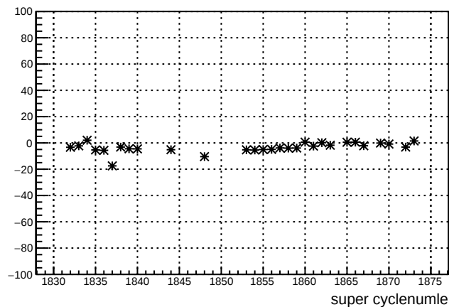
usl_11X12X : slug 39
