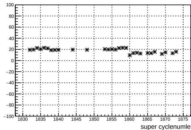
usr_4eY : slug 39
