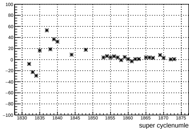
usr_4aY : slug 39
