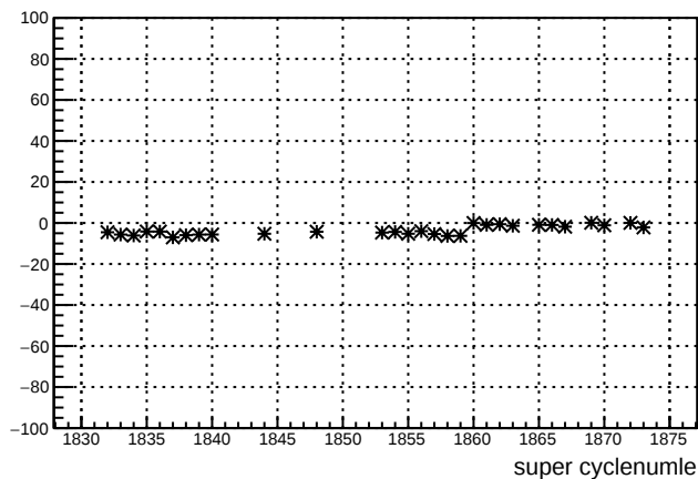
dsr_11X12X : slug 39
