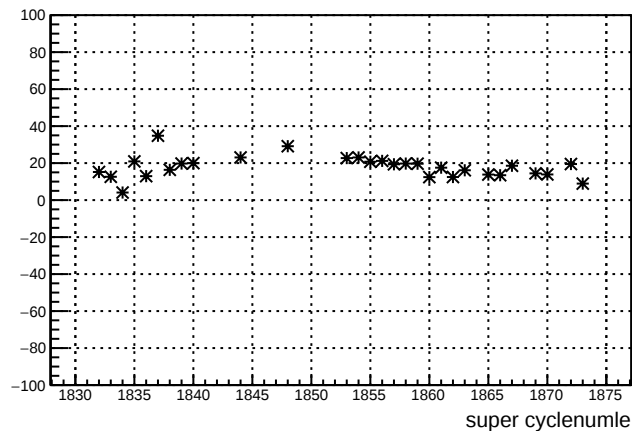
dsl_4eY : slug 39
