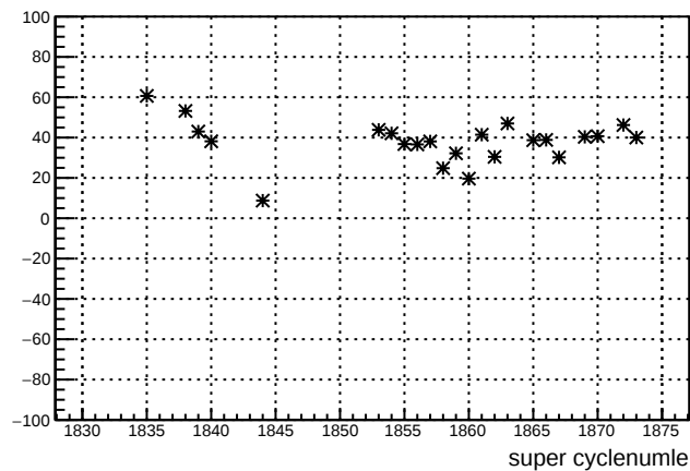
usl_4aY : slug 39
