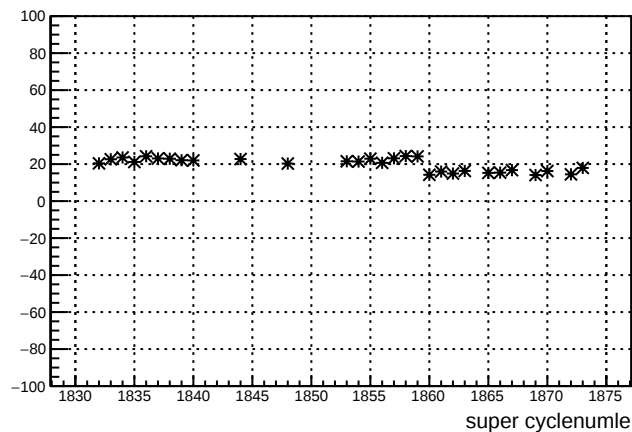
dsr_4eY : slug 39
