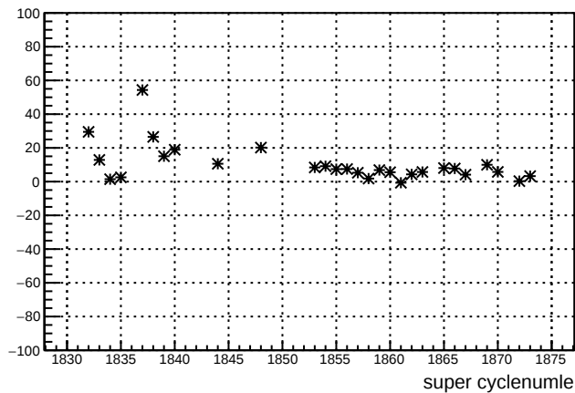
dsr_4aY : slug 39
