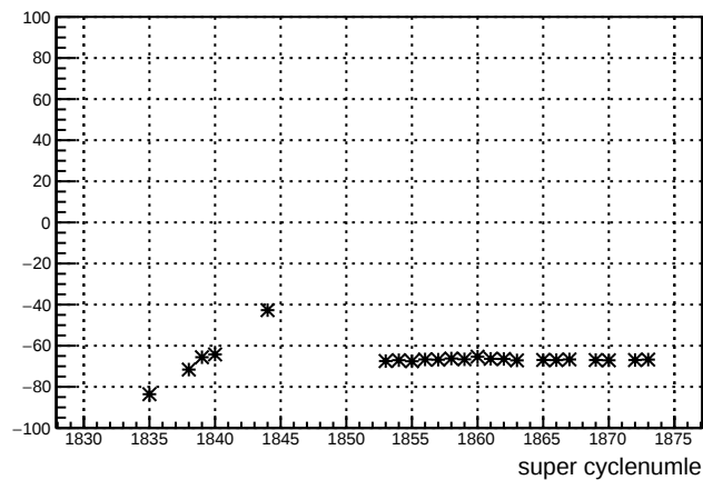
usl_4eY : slug 39
