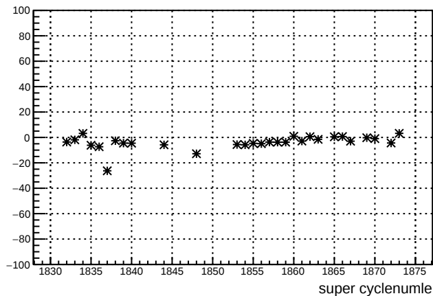
dsl_11X12X : slug 39
