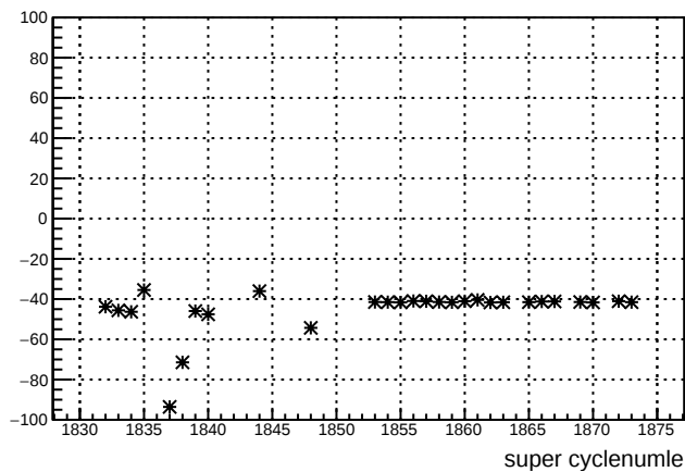
dsr_11X12X : slug 39
