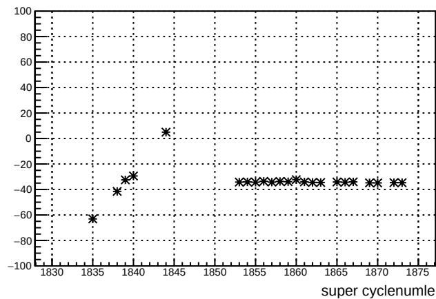
usl_11X12X : slug 39
