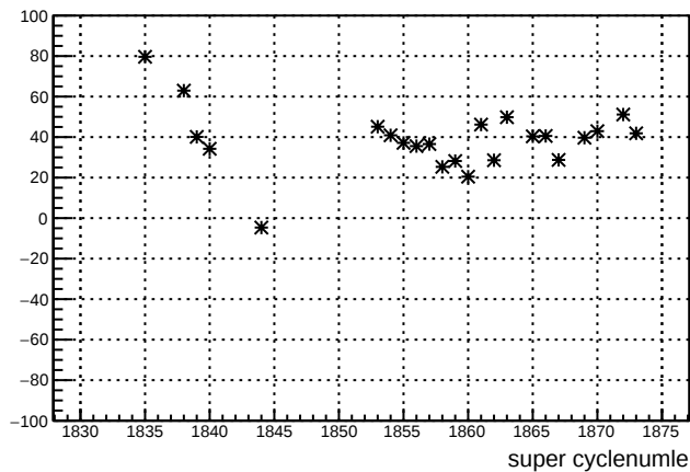
dsl_4aY : slug 39
